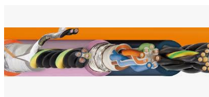
Leitungen für Bewegung: chainflex@ igus.de
