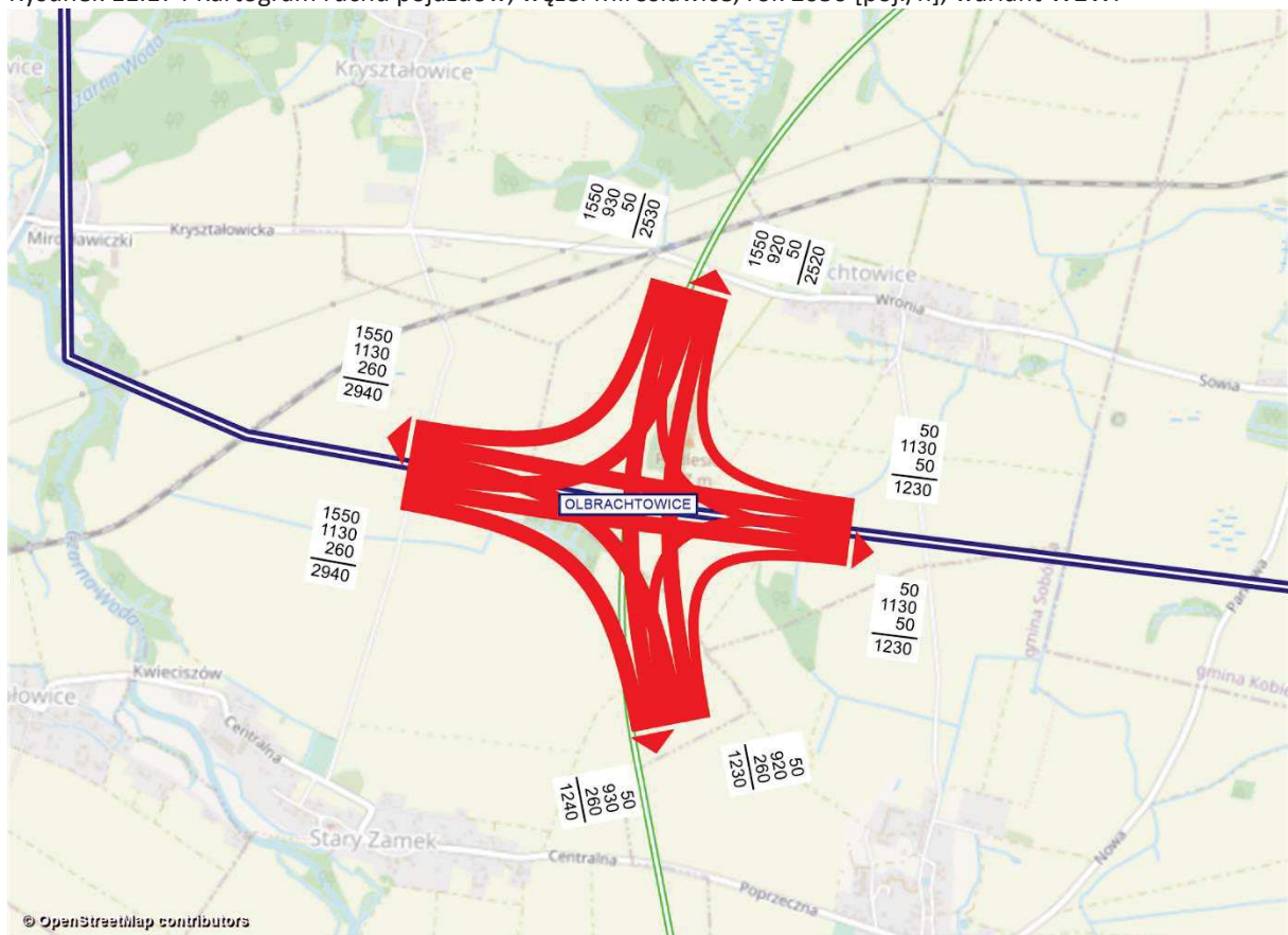
Rysunek 11.175 Kartogram ruchu pojazdów, węzeł Olbrachtowice, rok 2030 [poj./h], wariant W2W1
