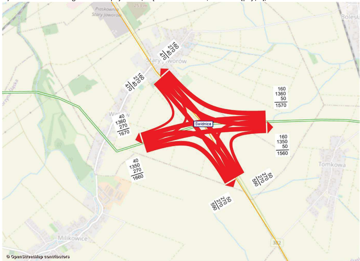
Rysunek 11.181 Kartogram ruchu pojazdów, węzeł Świdnica, rok 2030 [poj./h], wariant W2WI
