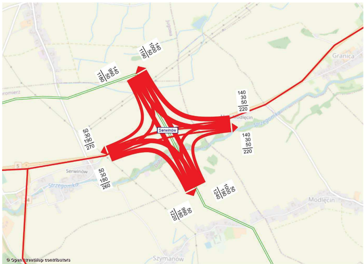
Rysunek 11.168 Kartogram ruchu pojazdów, węzeł Serwinów, rok 2030 [poj./h], wariant W1WIII
