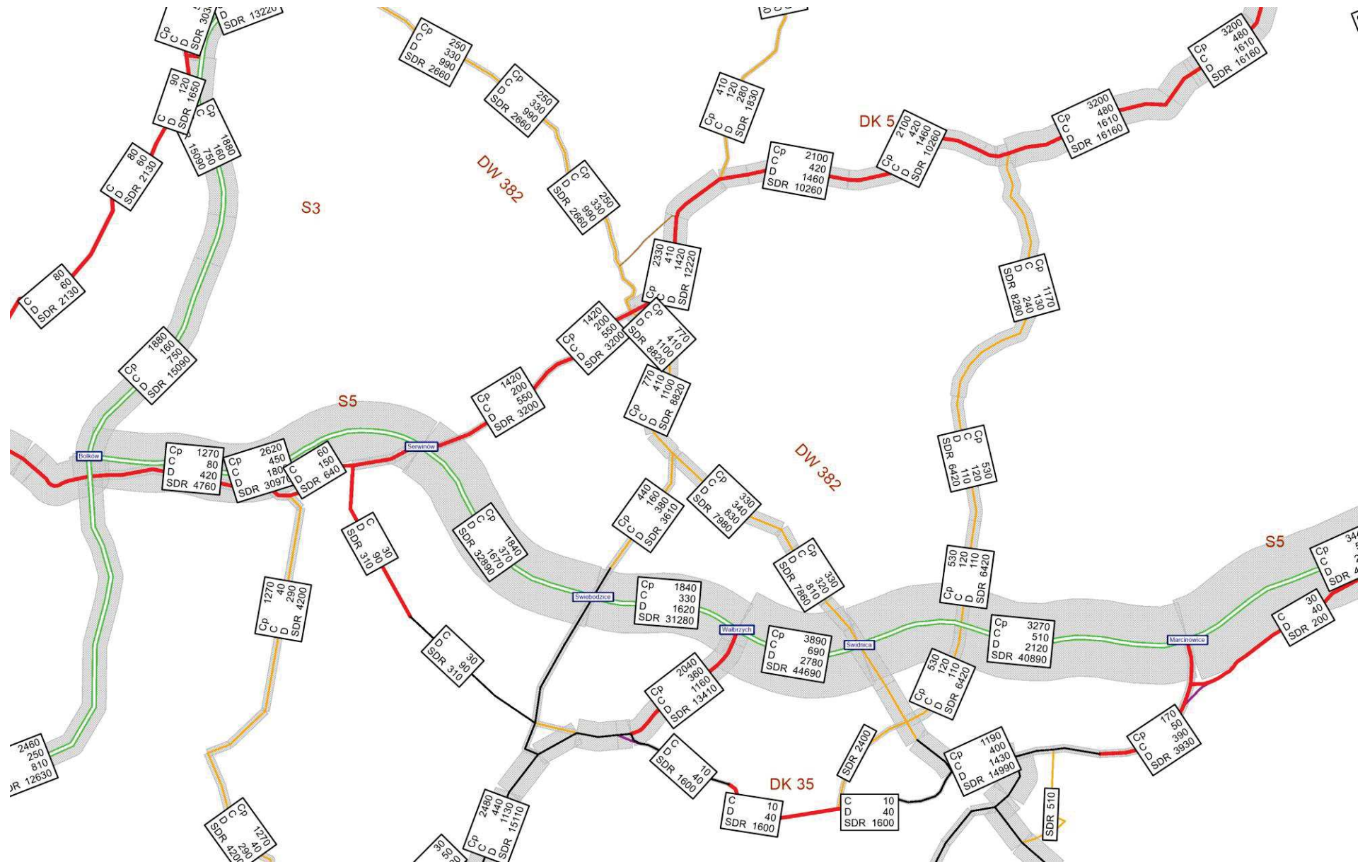
Rysunek 11.129 Natężenie pojazdów SDRR [poj./dobę], rok 2040 – W2.1WIII, rys 3
