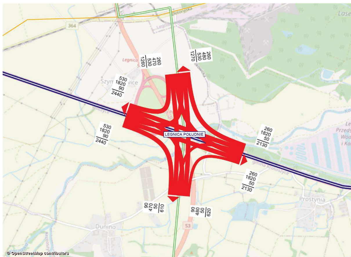
Rysunek 11.200 Kartogram ruchu pojazdów, węzeł Legnica Południe, rok 2030 [poj./h], wariant W2WIII
