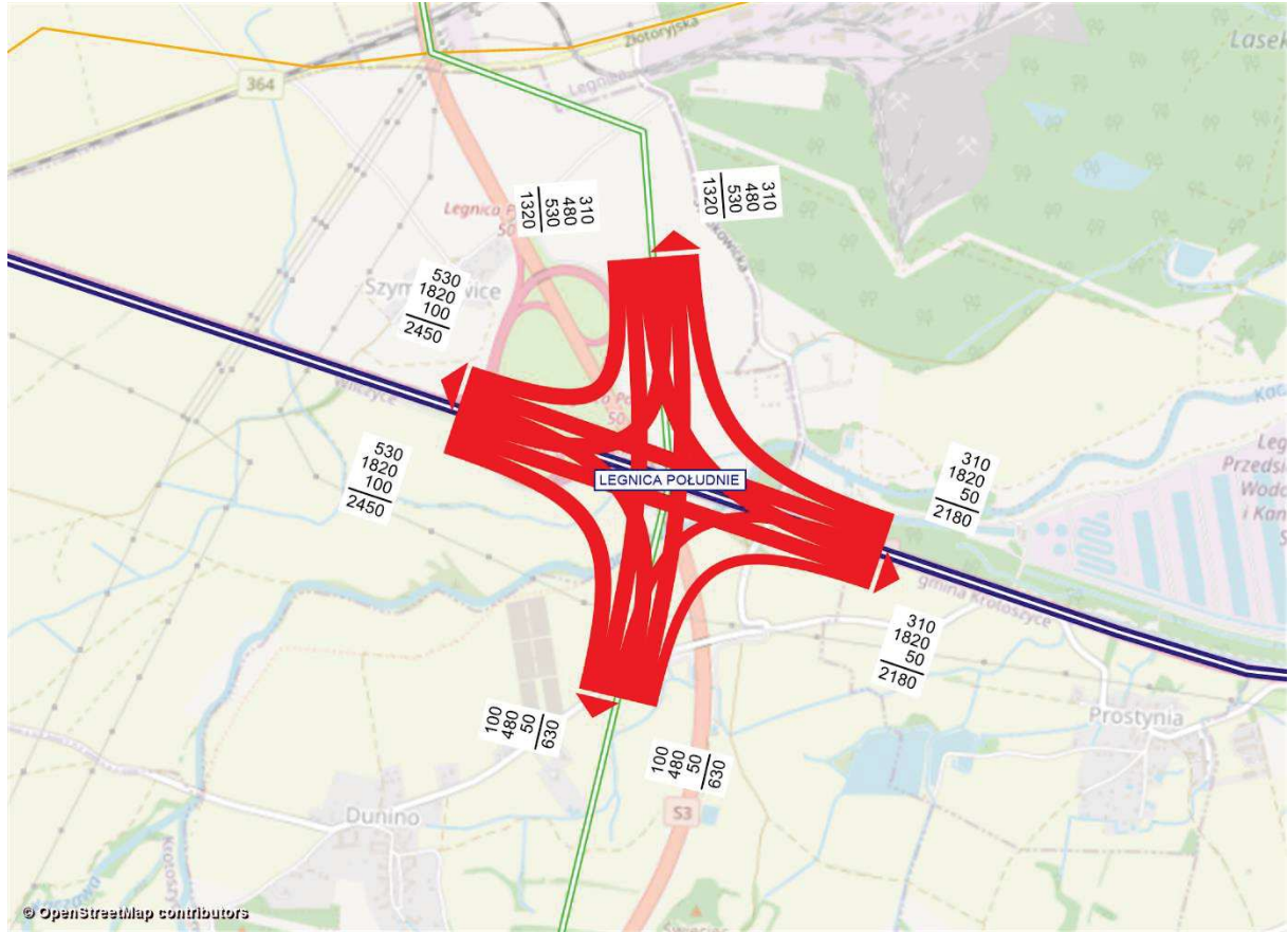
Rysunek 11.153 Kartogram ruchu pojazdów, węzeł Legnica Południe, rok 2030 [poj./h], wariant W1WIII
