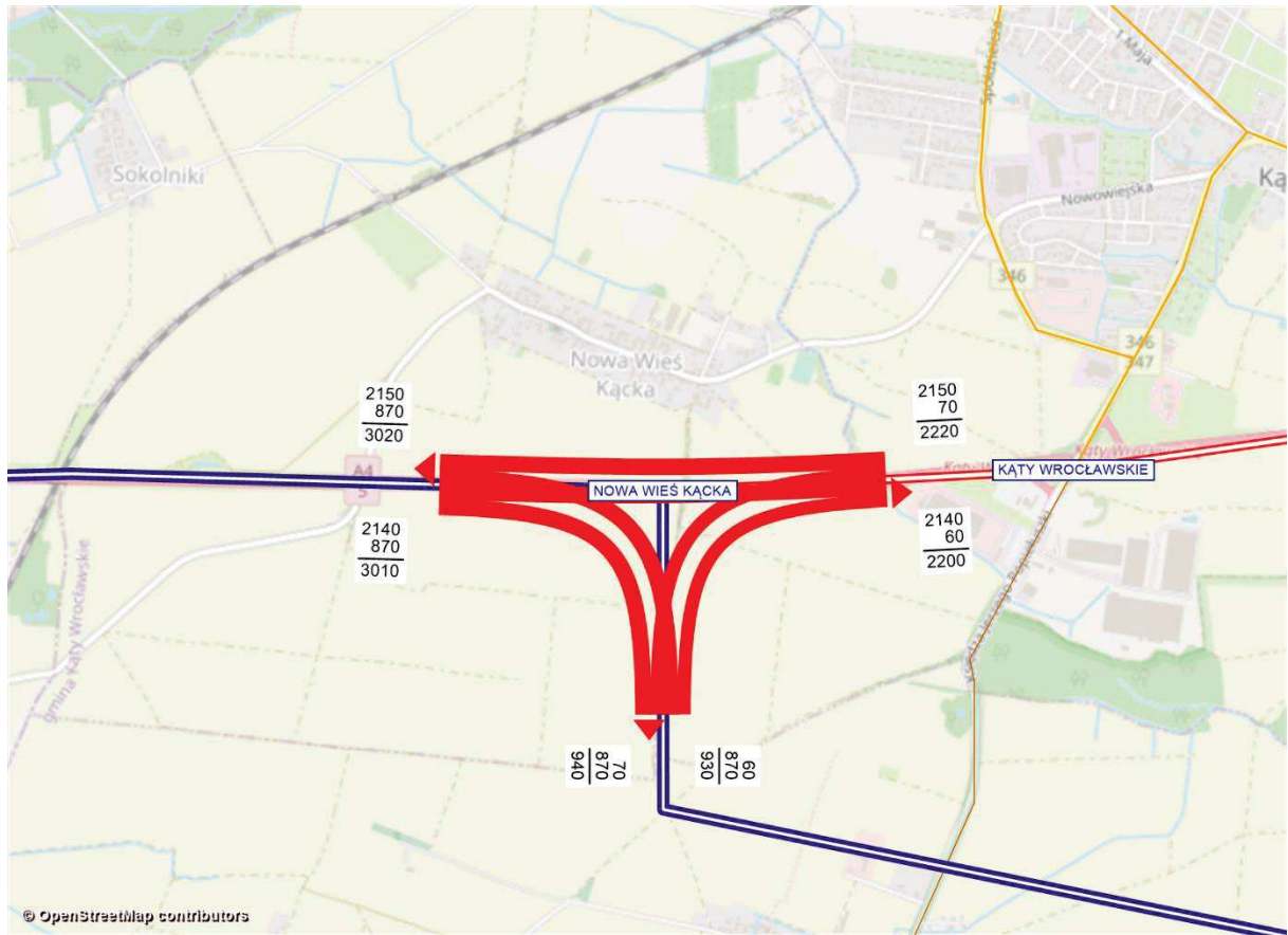
Rysunek 11.219 Kartogram ruchu pojazdów, węzeł Nowa Wieś Kącka, rok 2030 [poj./h], wariant W2.1W1
