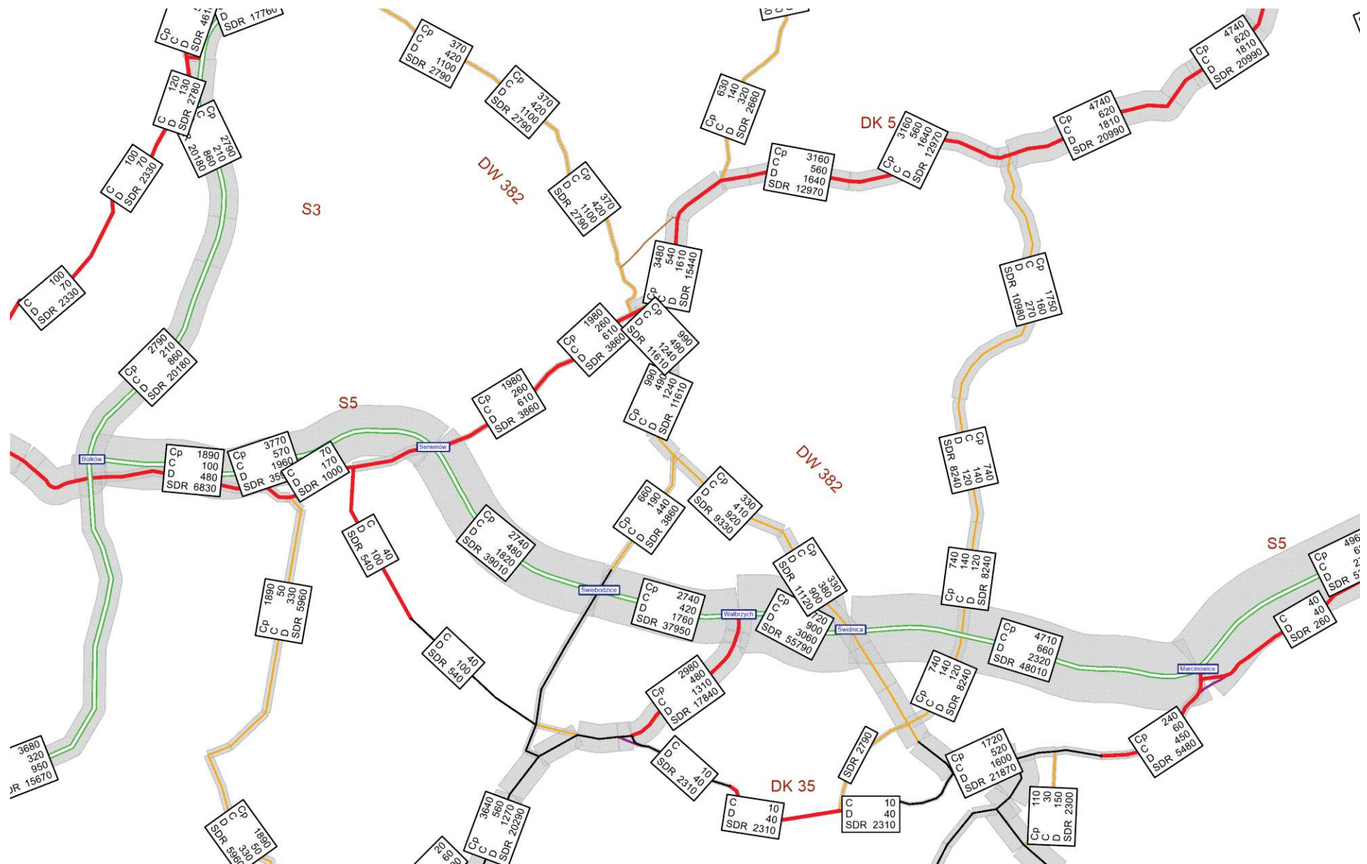
Rysunek 11.105 Natężenie pojazdów SDRR [poj./dobę], rok 2060 – W2.1WI, rys 3
