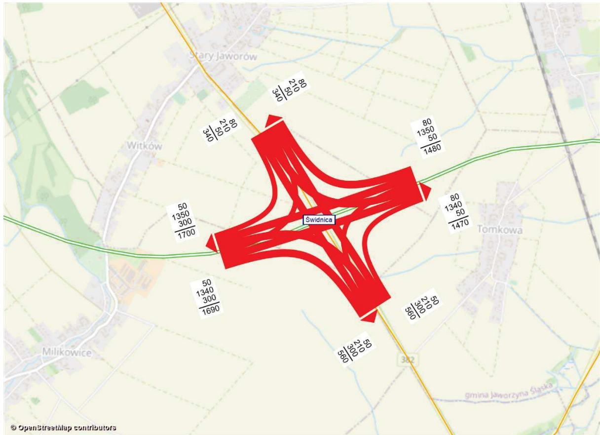
Rysunek 11.165 Kartogram ruchu pojazdów, węzeł Świdnica, rok 2030 [poj./h], wariant W1WIII
