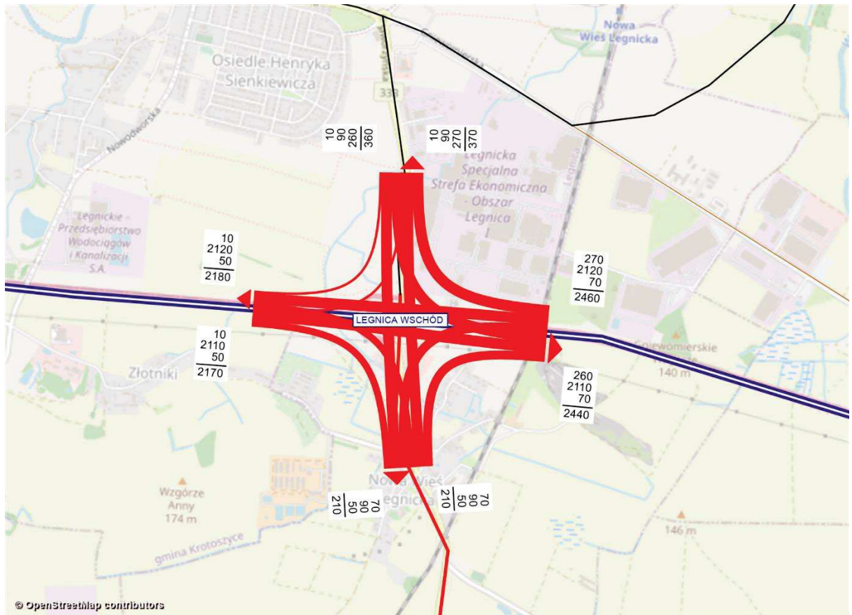
Rysunek 11.154 Kartogram ruchu pojazdów, węzeł Legnica Wschód, rok 2030 [poj./h], wariant W1WIII
