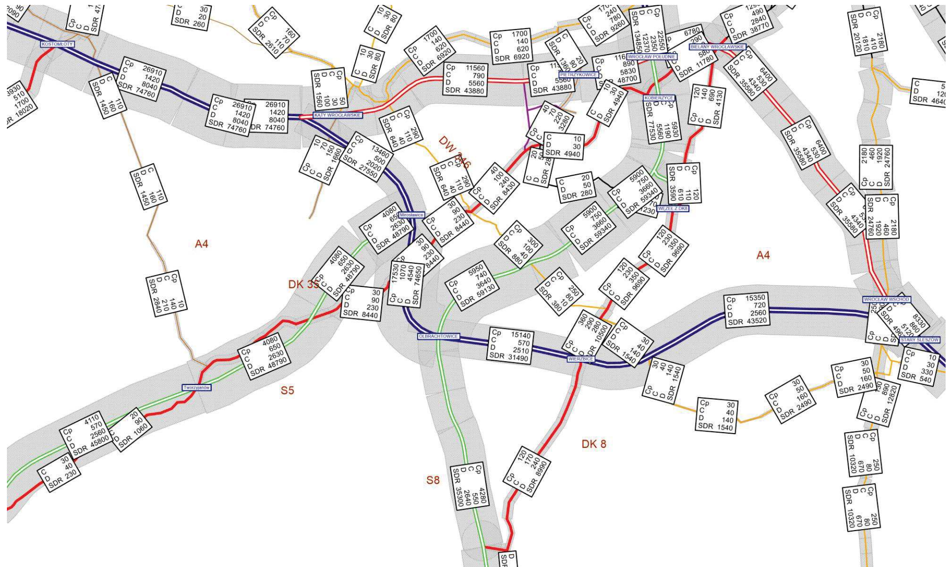
Rysunek 11.101 Natężenie pojazdów SDRR [poj./dobę], rok 2050 – W2.1WI, rys 2
