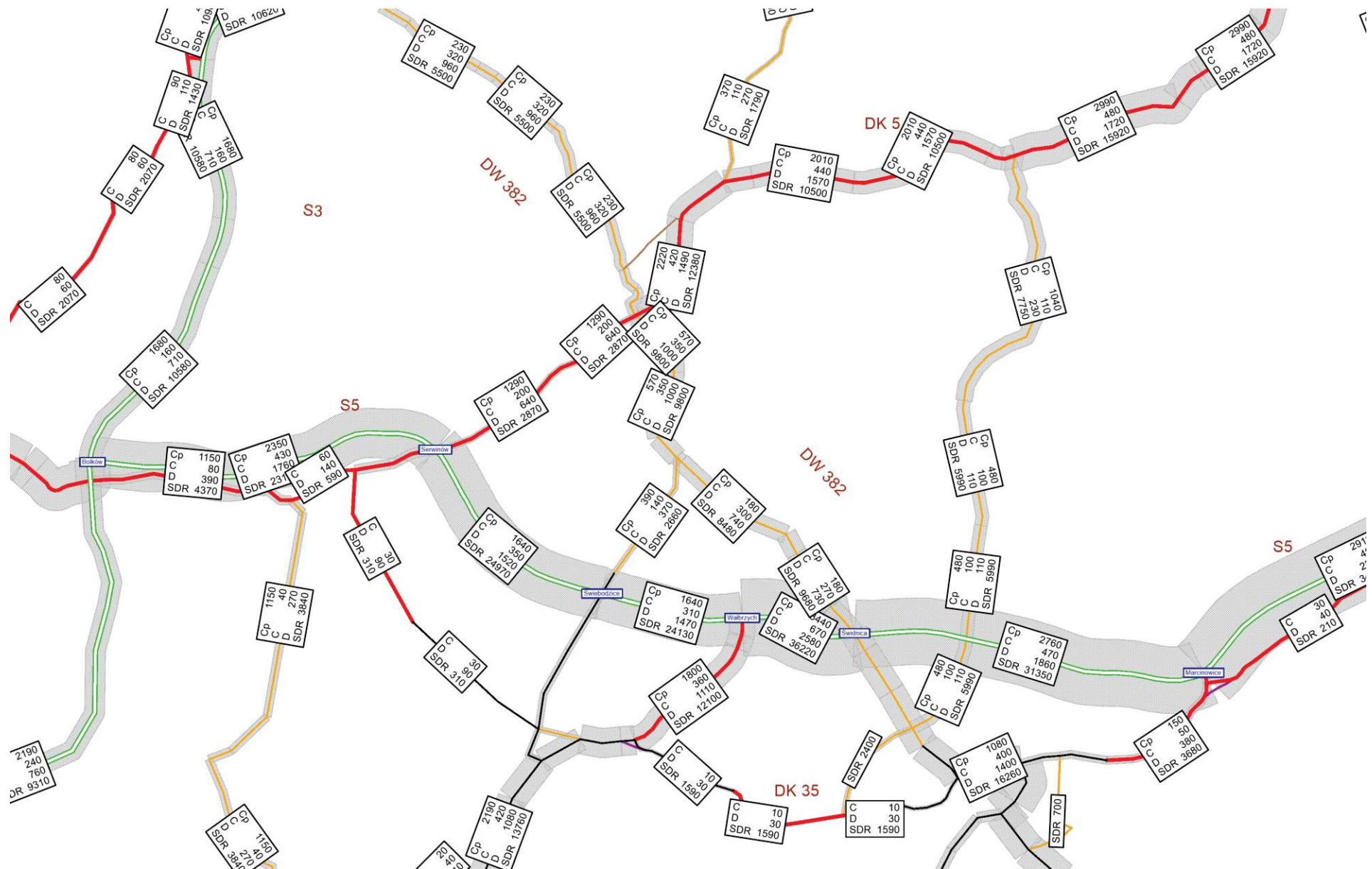
Rysunek 11.96 Natężenie pojazdów SDRR [poj./dobę], rok 2035 – W2.1WI, rys 3
