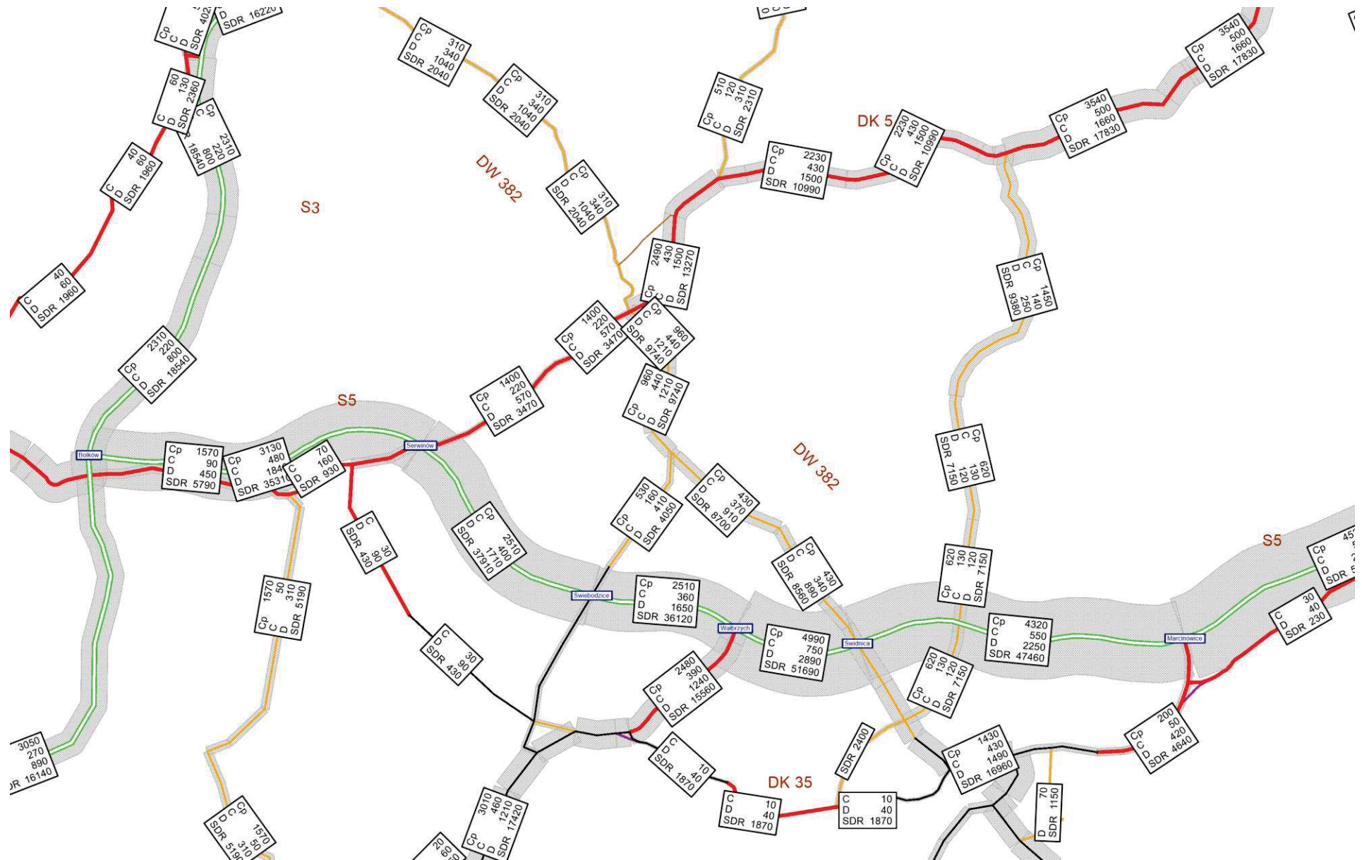
Rysunek 11.132 Natężenie pojazdów SDRR [poj./dobę], rok 2050 – W2.1WIII, rys 3
