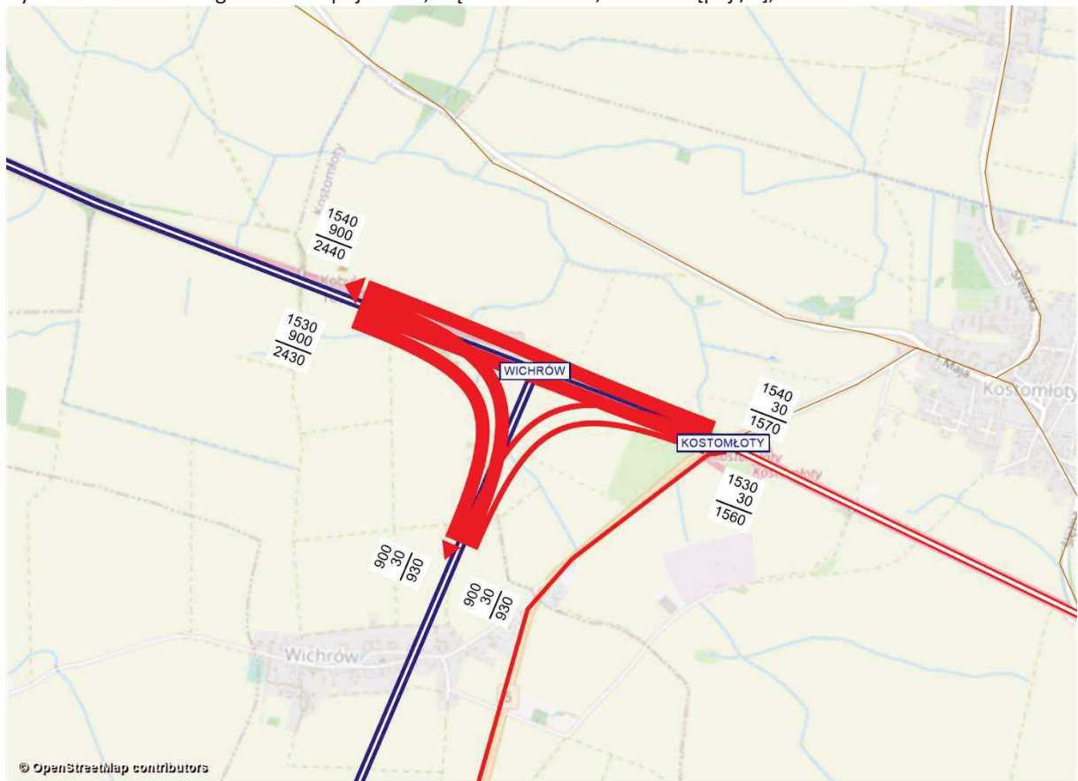
Rysunek 11.173 Kartogram ruchu pojazdów, węzeł Wichrów, rok 2030 [poj./h], wariant W2W1
