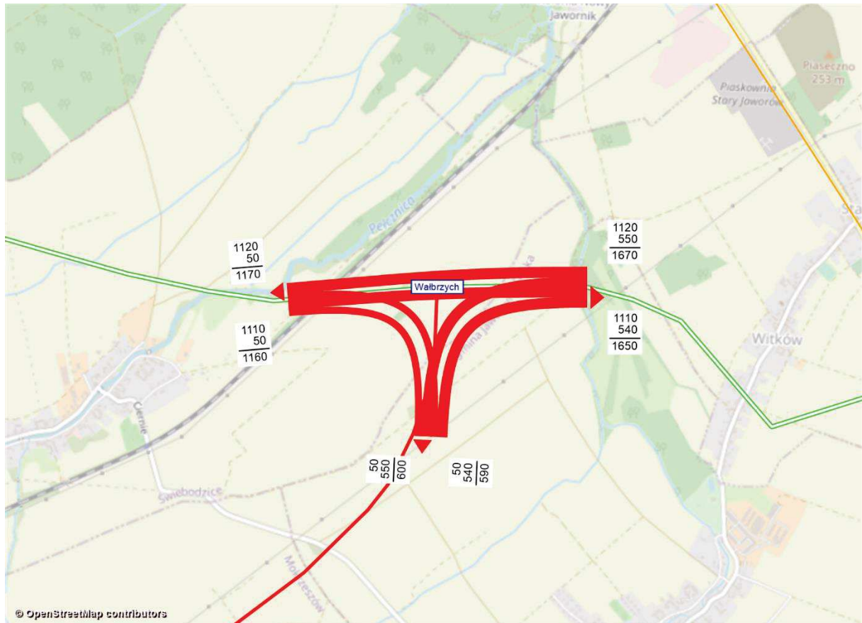
Rysunek 11.182 Kartogram ruchu pojazdów, węzeł Wałbrzych, rok 2030 [poj./h], wariant W2W1
