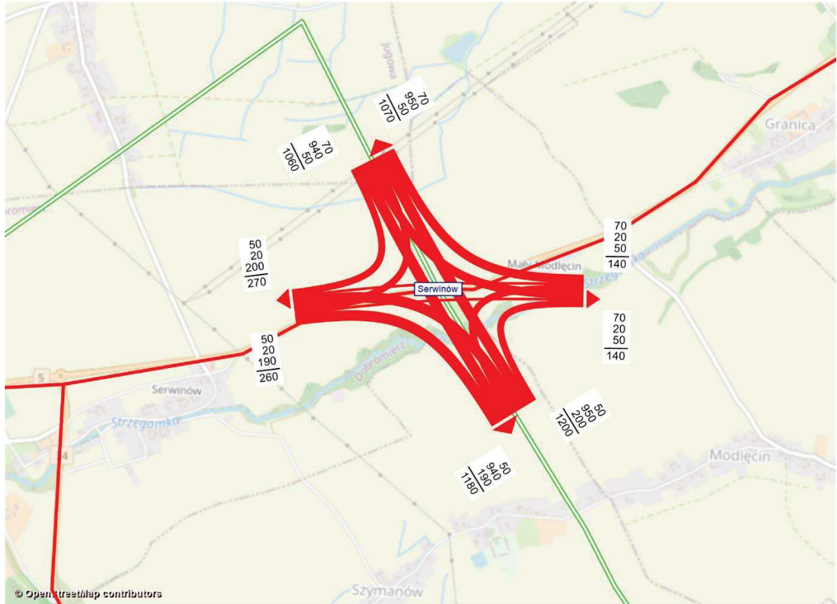
Rysunek 11.184 Kartogram ruchu pojazdów, węzeł Serwinów, rok 2030 [poj./h], wariant W2WI
