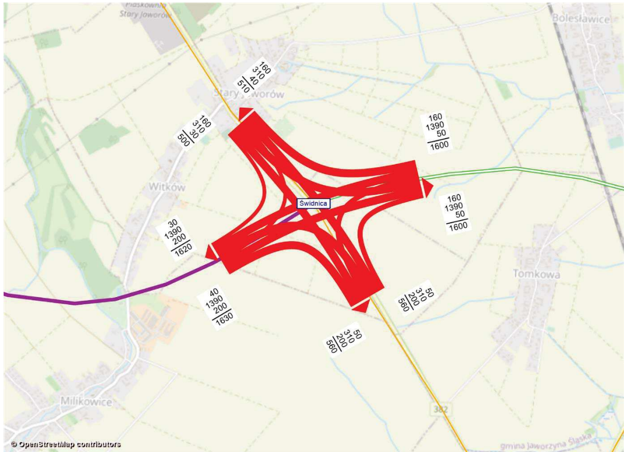
Rysunek 11.148 Kartogram ruchu pojazdów, węzeł Świdnica, rok 2030 [poj./h], wariant W1WII
