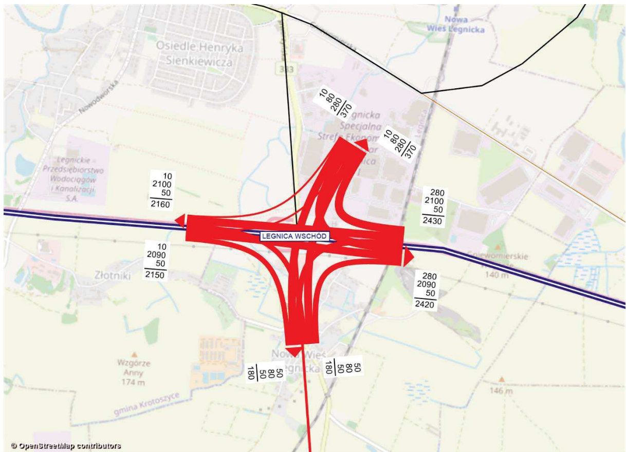
Rysunek 11.233 Kartogram ruchu pojazdów, węzeł Legnica Wschód, rok 2030 [poj./h], wariant W2.1WII
