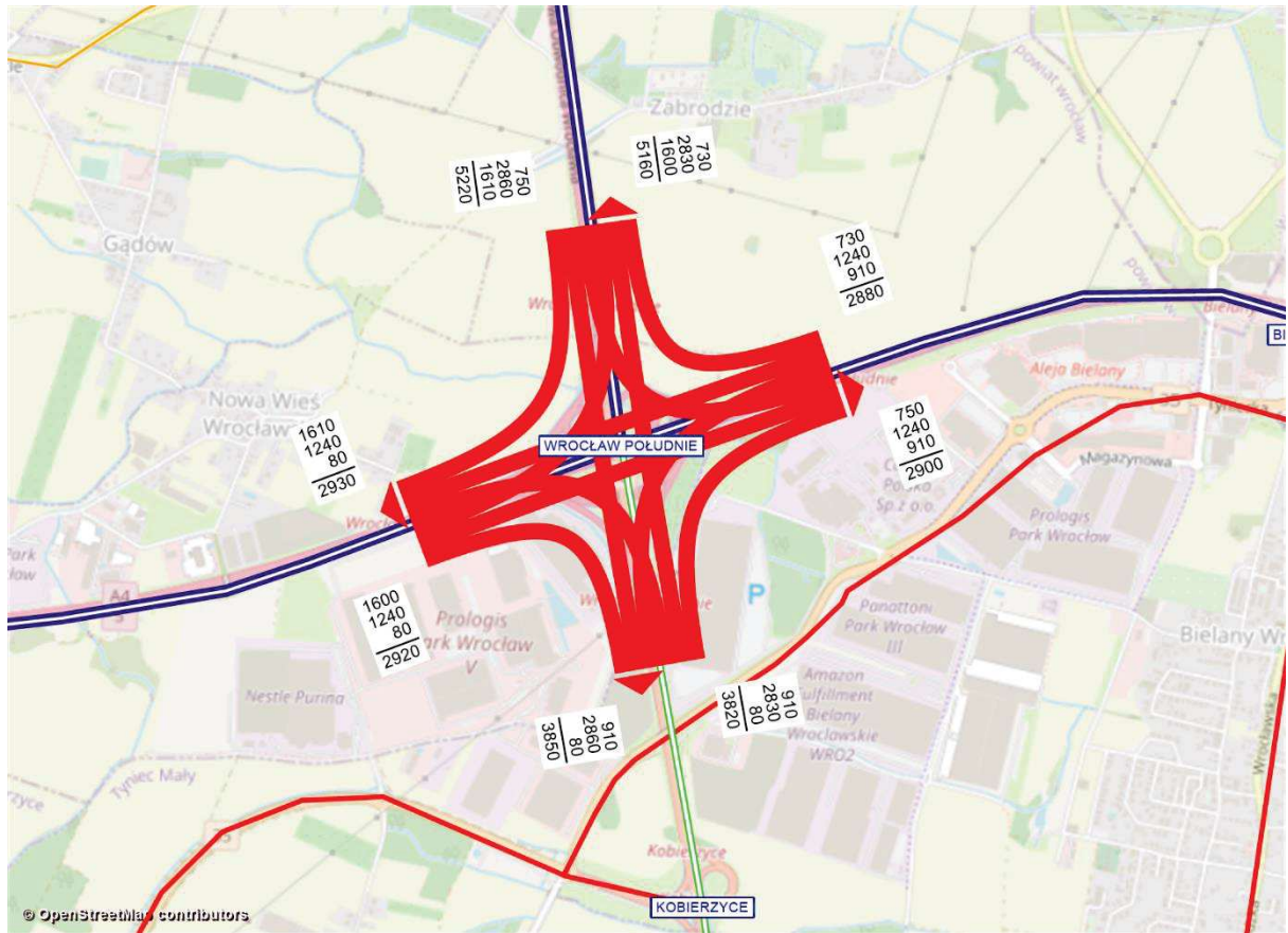
Rysunek 11.142 Kartogram ruchu pojazdów, węzeł Wrocław Południe, rok 2030 [poj./h], wariant W1WII
