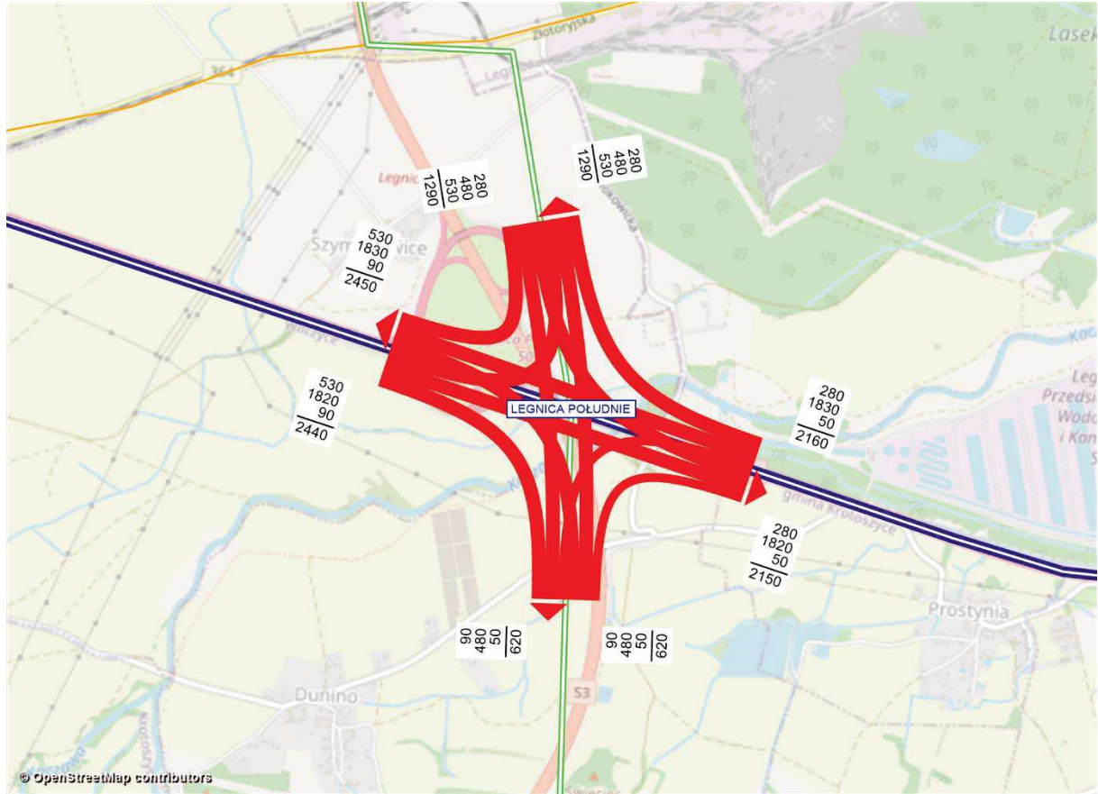
Rysunek 11.215 Kartogram ruchu pojazdów, węzeł Legnica Południe, rok 2030 [poj./h], wariant W2.1W1
