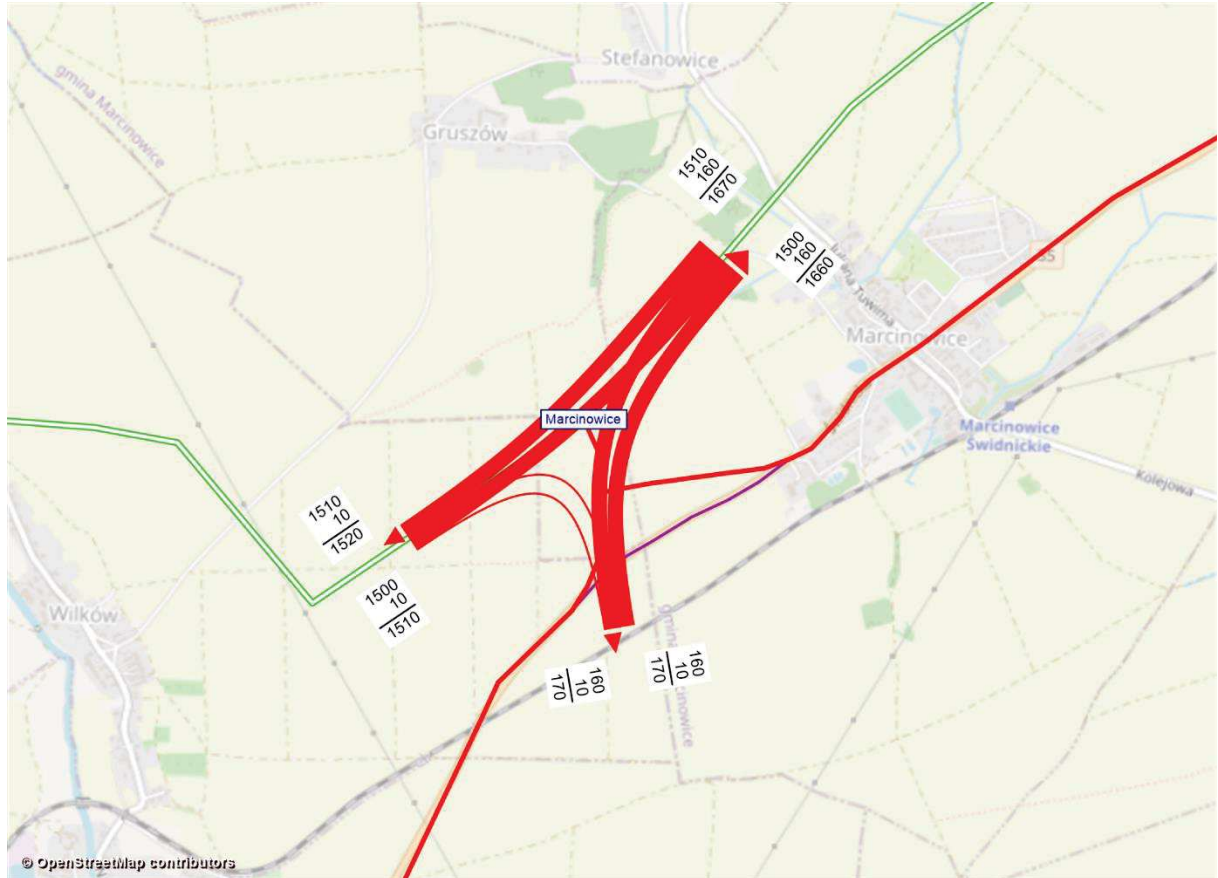
Rysunek 11.180 Kartogram ruchu pojazdów, węzeł Marcinowice, rok 2030 [poj./h], wariant W2WI
