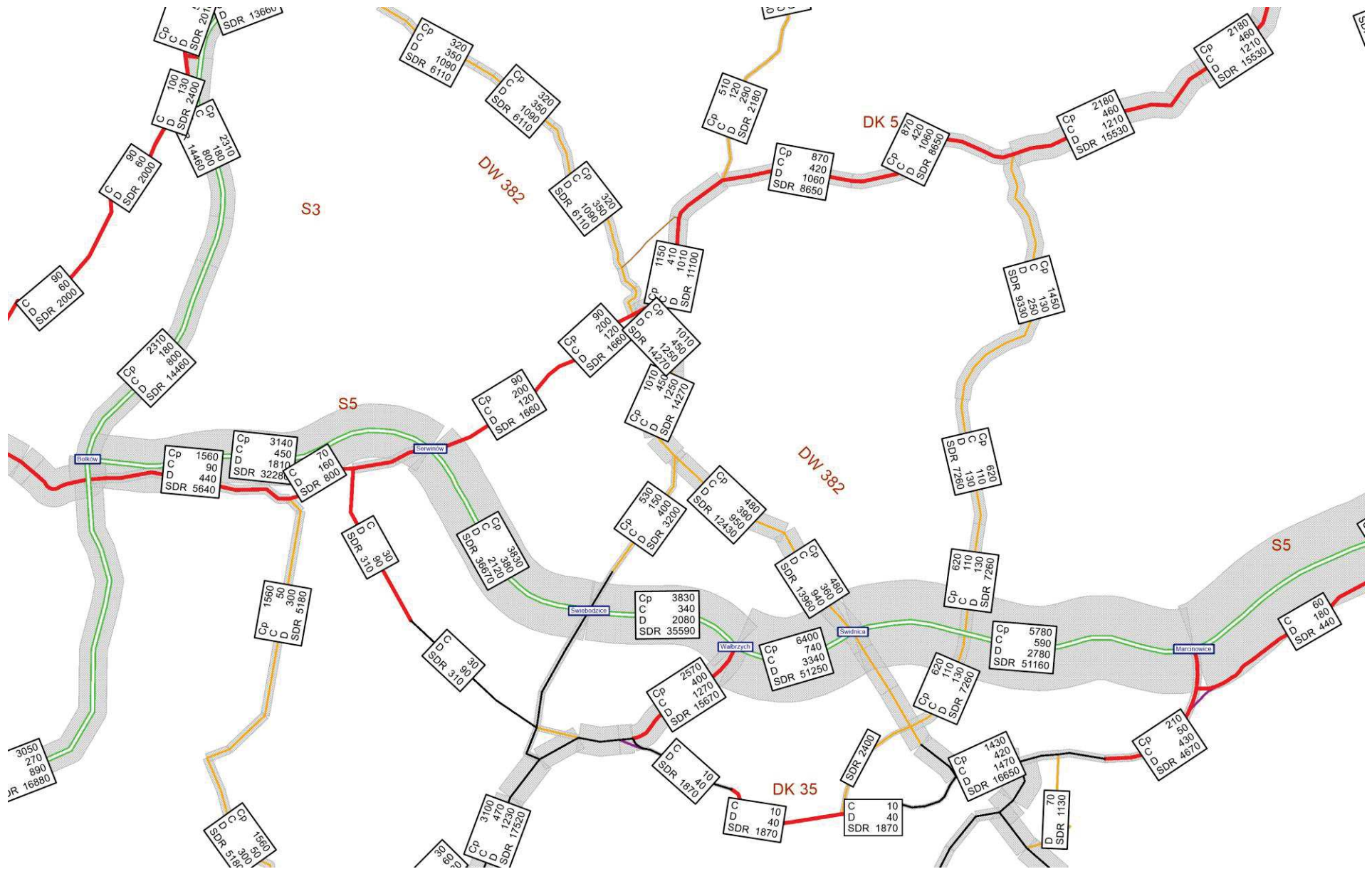
Rysunek 11.117 Natężenie pojazdów SDRR [poj./dobę], rok 2050 – W2.1WII, rys 3
