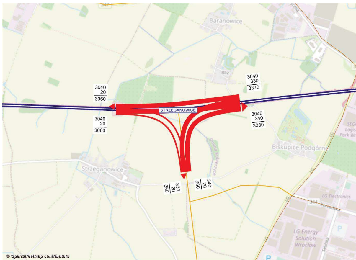
Rysunek 11.158 Kartogram ruchu pojazdów, węzeł Strzegánowice, rok 2030 [poj./h], wariant W1WIII
