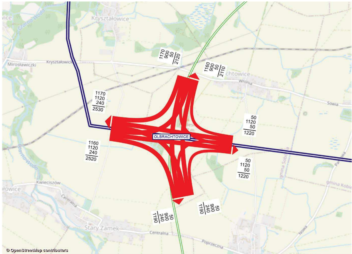
Rysunek 11.221 Kartogram ruchu pojazdów, węzeł Olbrachtowice, rok 2030 [poj./h], wariant W2.1W1
