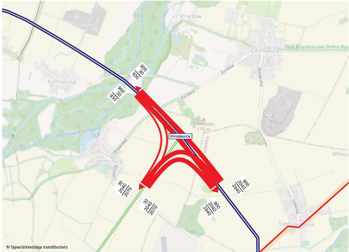
Rysunek 11.178 Kartogram ruchu pojazdów, węzeł Mirosławice, rok 2030 [poj./h], wariant W2W1
