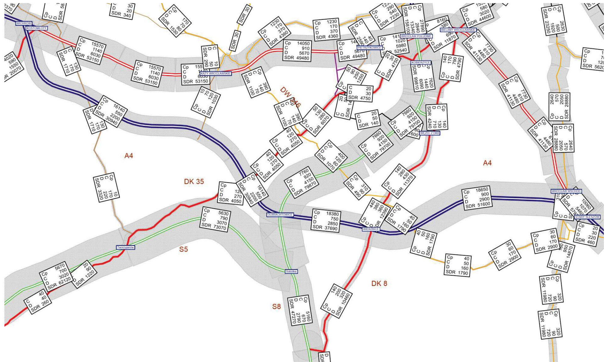
Rysunek 11.89 Natężenie pojazdów SDRR [poj./dobę], rok 2060 – WZVIII, rys 2
