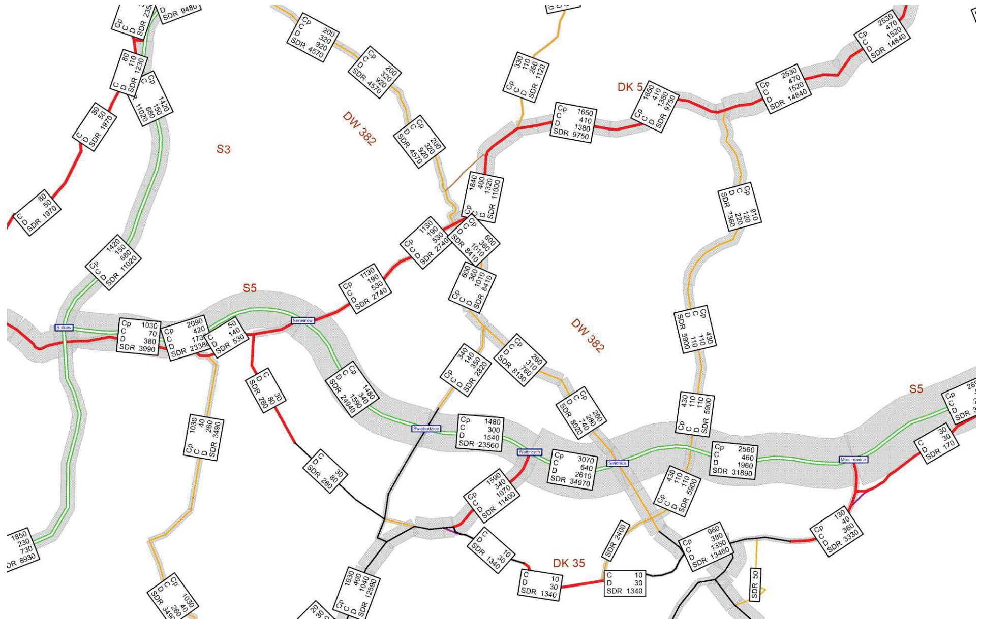
Rysunek 11.123 Natężenie pojazdów SDRR [poj./dobę], rok 2030 – W2.1WIII, rys 3
