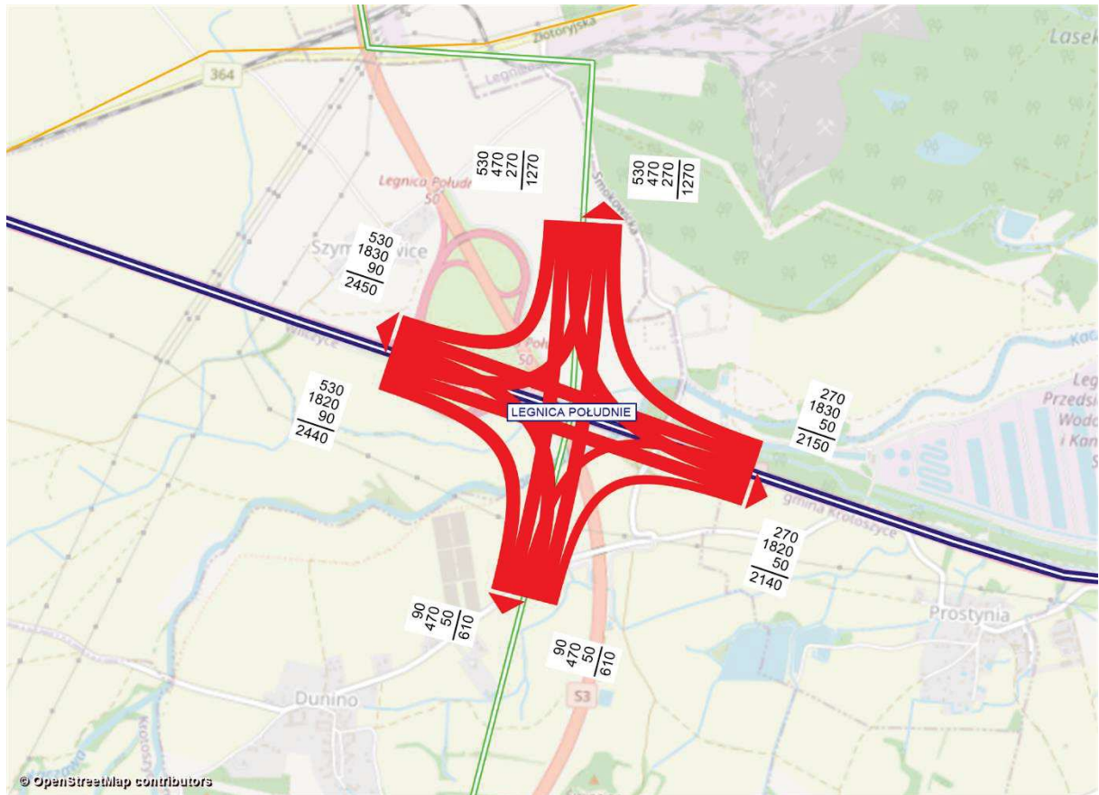
Rysunek 11.170 Kartogram ruchu pojazdów, węzeł Legnica Południe, rok 2030 [poj./h], wariant W2WI
