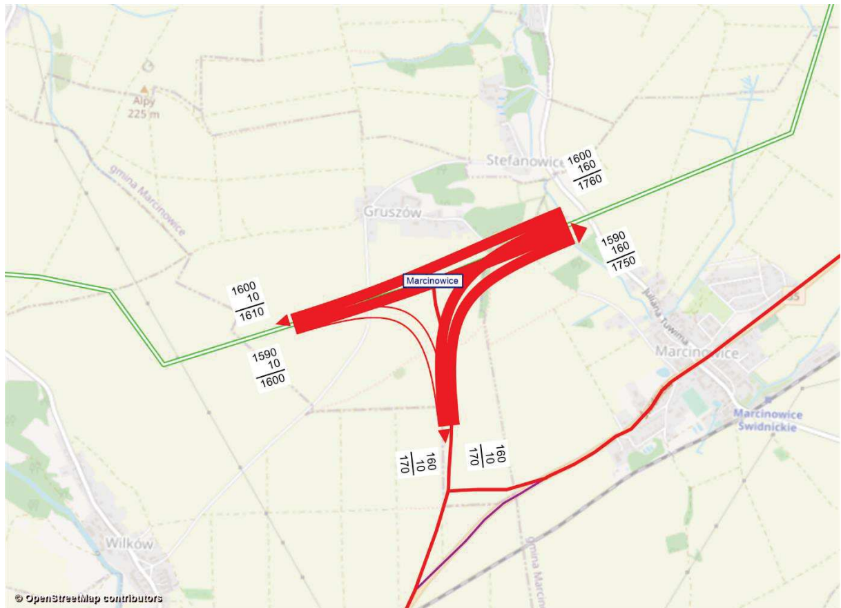
Rysunek 11.209 Kartogram ruchu pojazdów, węzeł Marcinowice, rok 2030 [poj./h], wariant W2WIII
