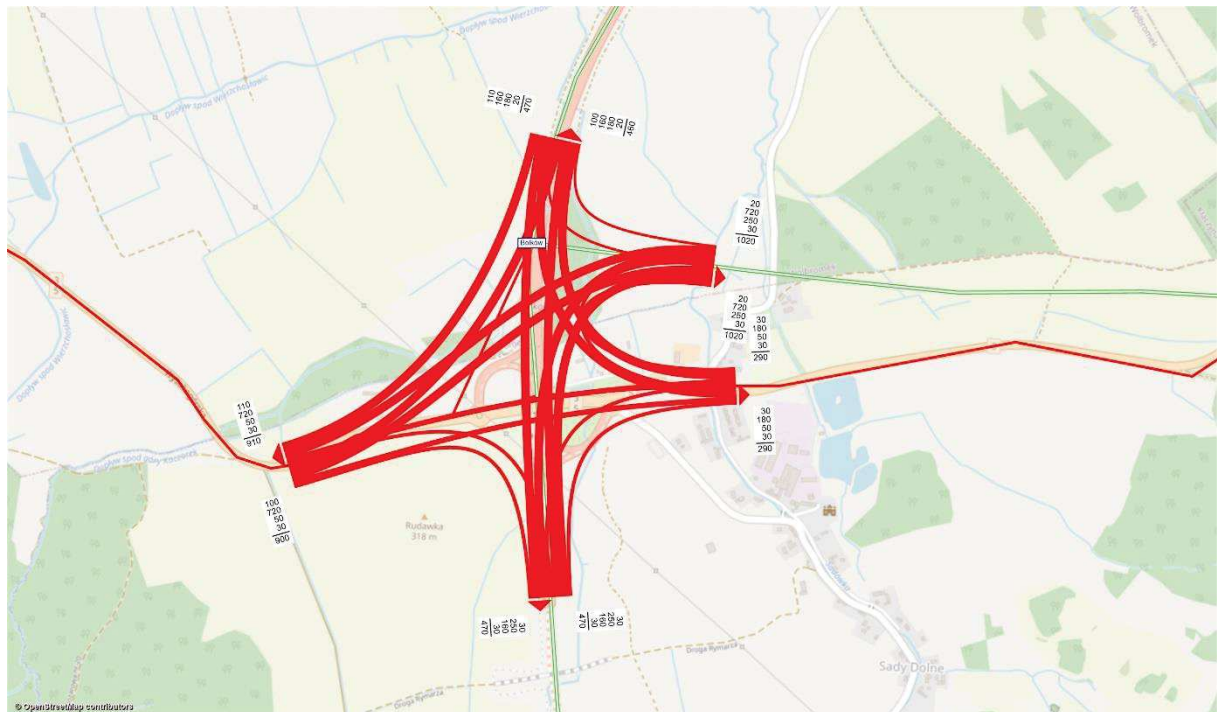
Rysunek 11.185 Kartogram ruchu pojazdów, węzeł Bolków, rok 2030 [poj./h], wariant W2WI
