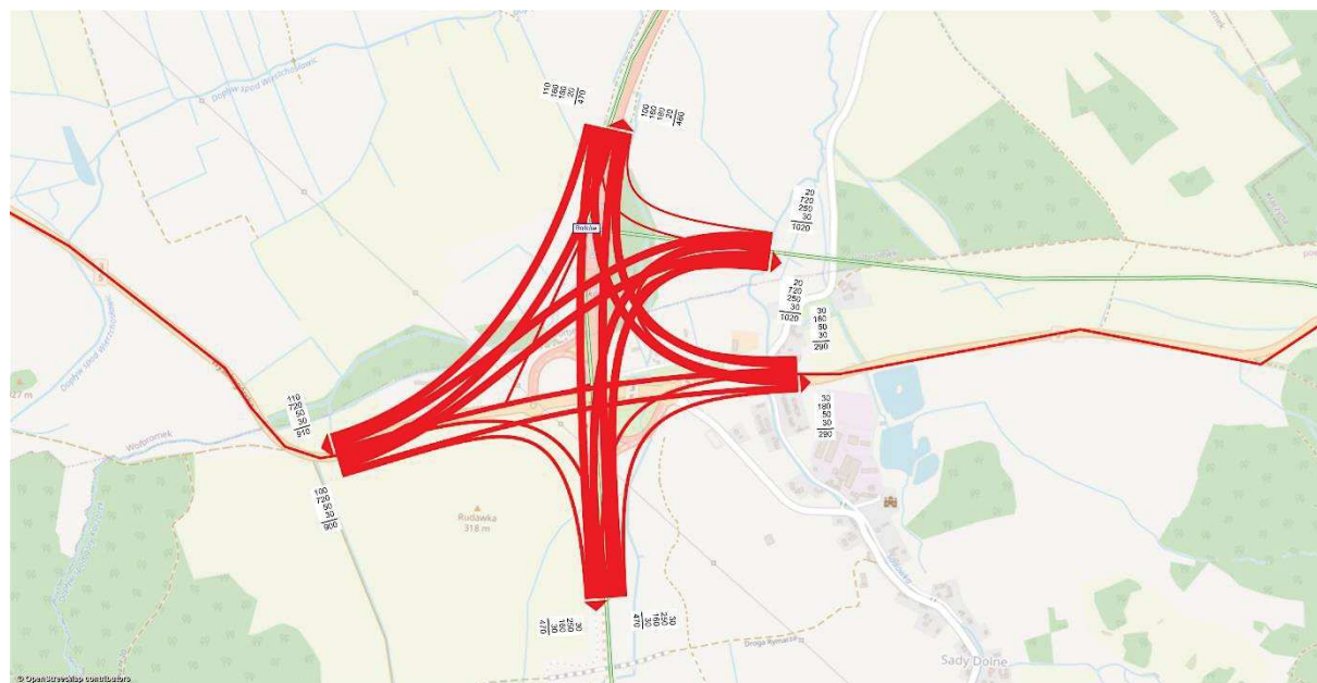
Rysunek 11.231 Kartogram ruchu pojazdów, węzeł Bolków, rok 2030 [poj./h], wariant W2.1W1
