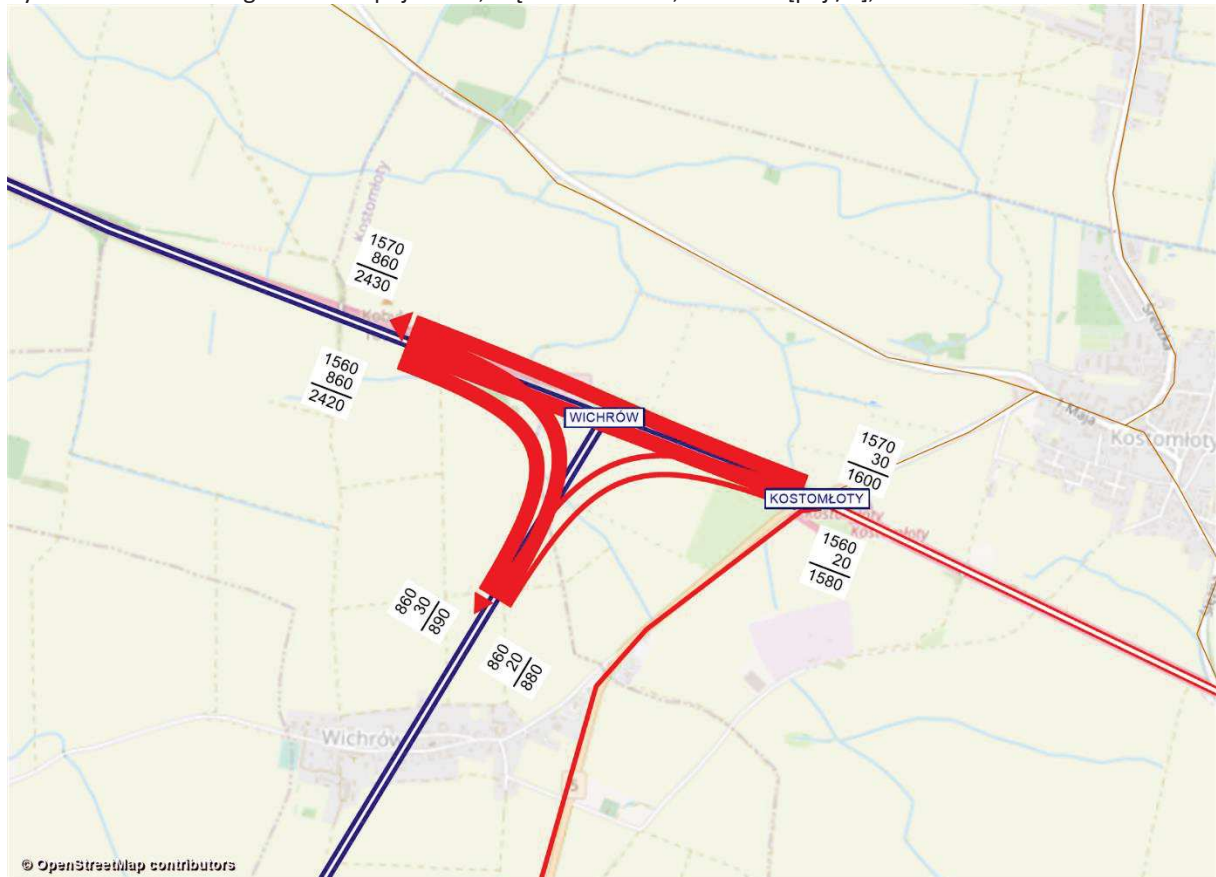
Rysunek 11.189 Kartogram ruchu pojazdów, węzeł Wichrów, rok 2030 [poj./h], wariant W2WII
