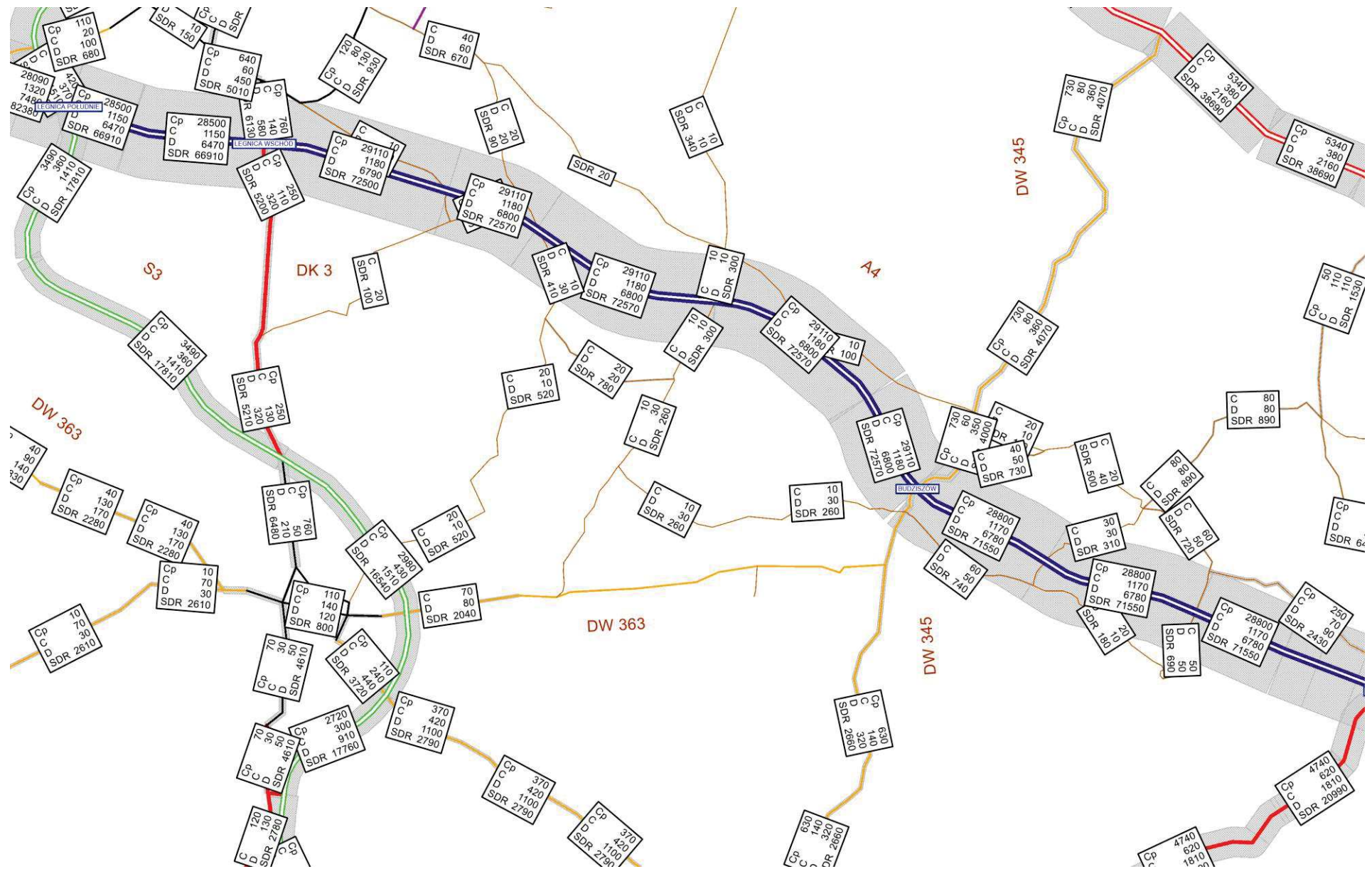
Rysunek 11.103 Natężenie pojazdów SDRR [poj./dobę], rok 2060 – W2.1WI, rys 1
