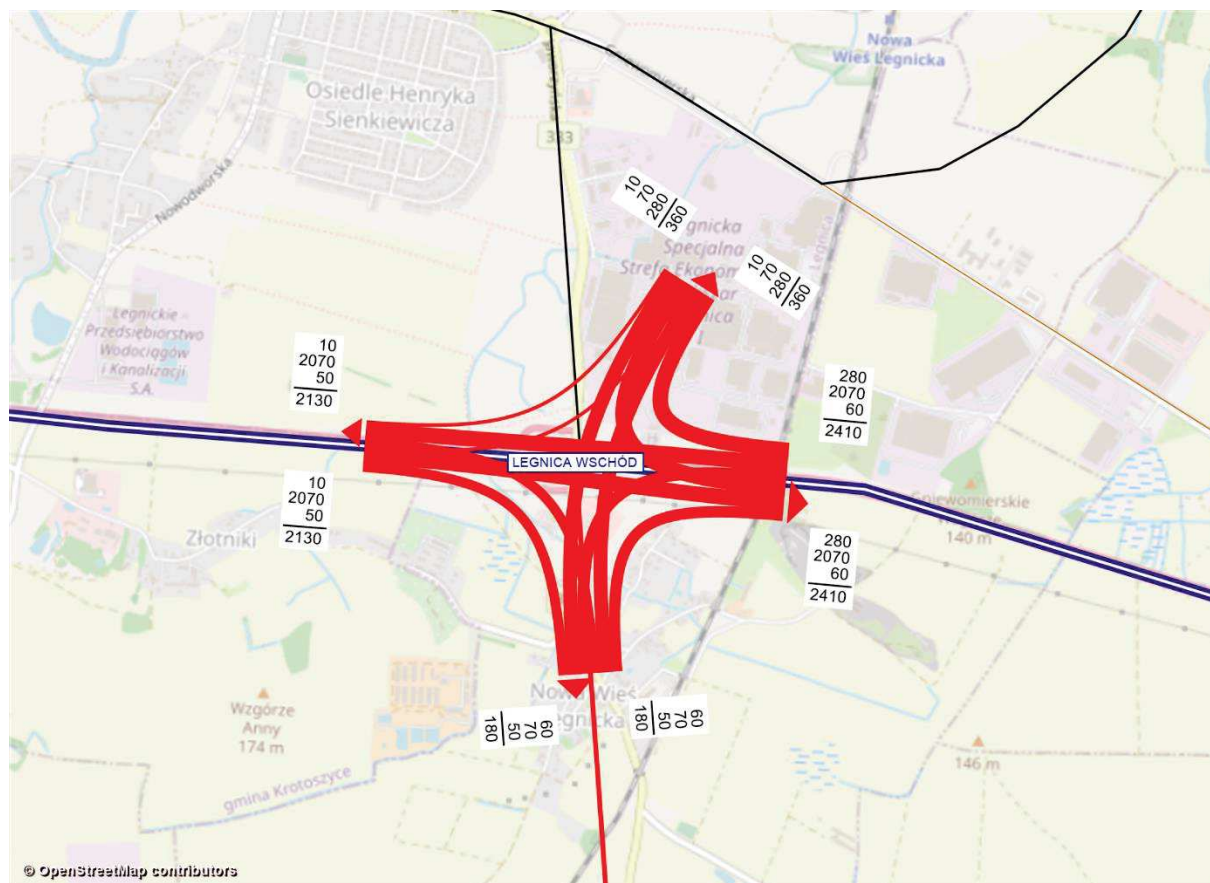
Rysunek 11.201 Kartogram ruchu pojazdów, węzeł Legnica Wschód, rok 2030 [poj./h], wariant W2WIII
