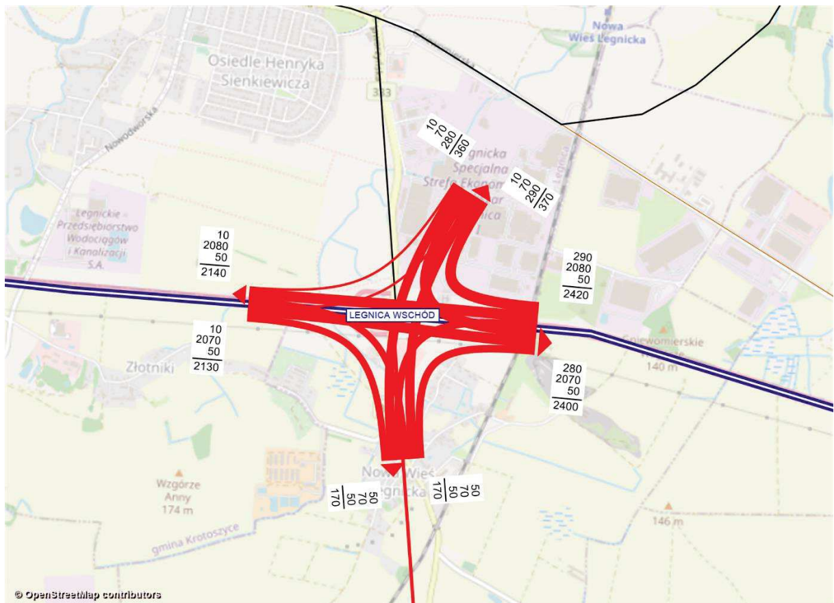
Rysunek 11.187 Kartogram ruchu pojazdów, węzeł Legnica Wschód, rok 2030 [poj./h], wariant W2WII
