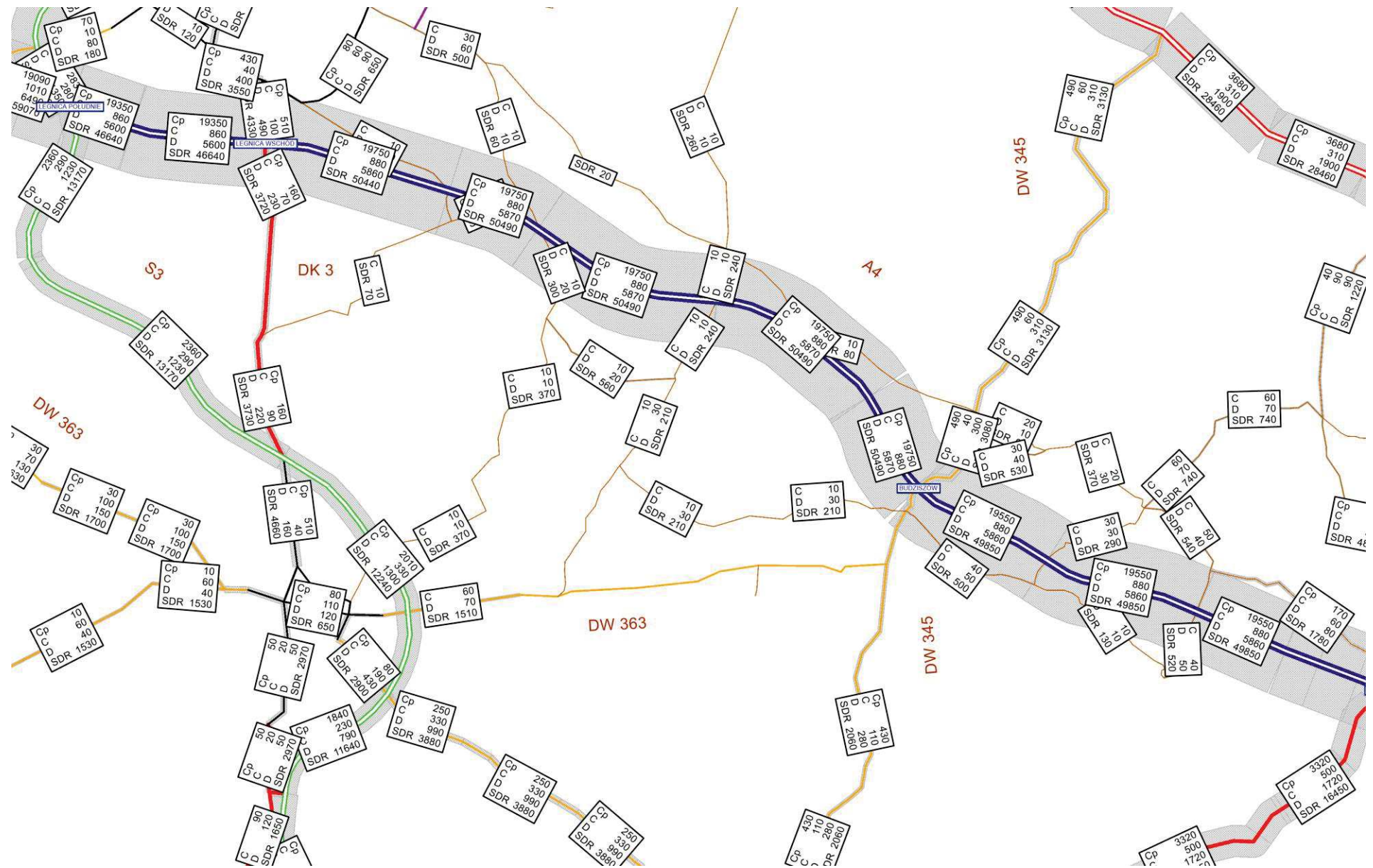
Rysunek 11.97 Natężenie pojazdów SDRR [poj./dobę], rok 2040 – W2.1WI , rys 1
