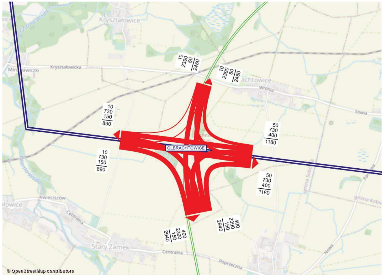
Rysunek 11.204 Kartogram ruchu pojazdów, węzeł Olbrachtwice, rok 2030 [poj./h], wariant W2WIII
