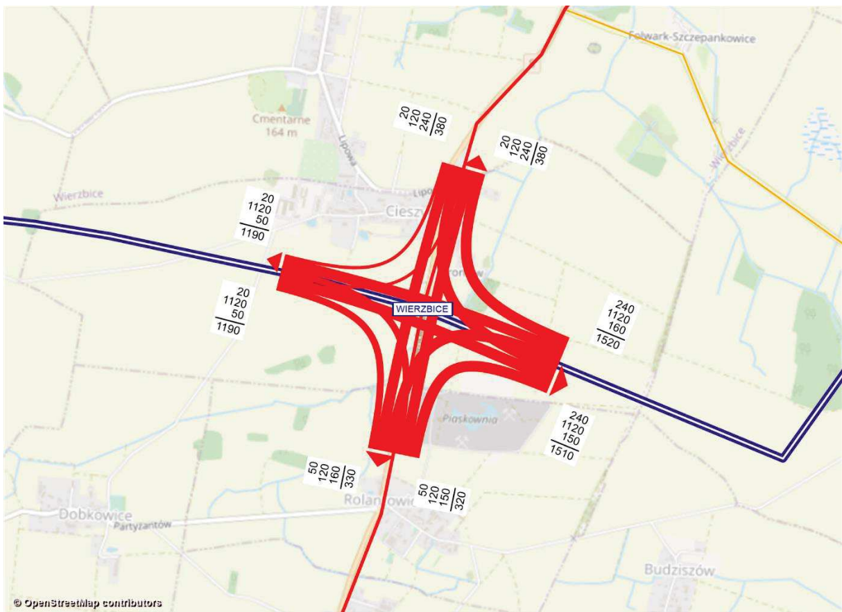
Rysunek 11.191 Kartogram ruchu pojazdów, węzeł Wierzbice, rok 2030 [poj./h], wariant W2WII
