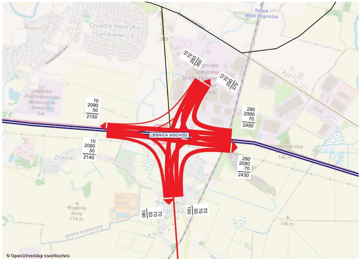
Rysunek 11.171 Kartogram ruchu pojazdów, węzeł Legnica Wschód, rok 2030 [poj./h], wariant W2WI
