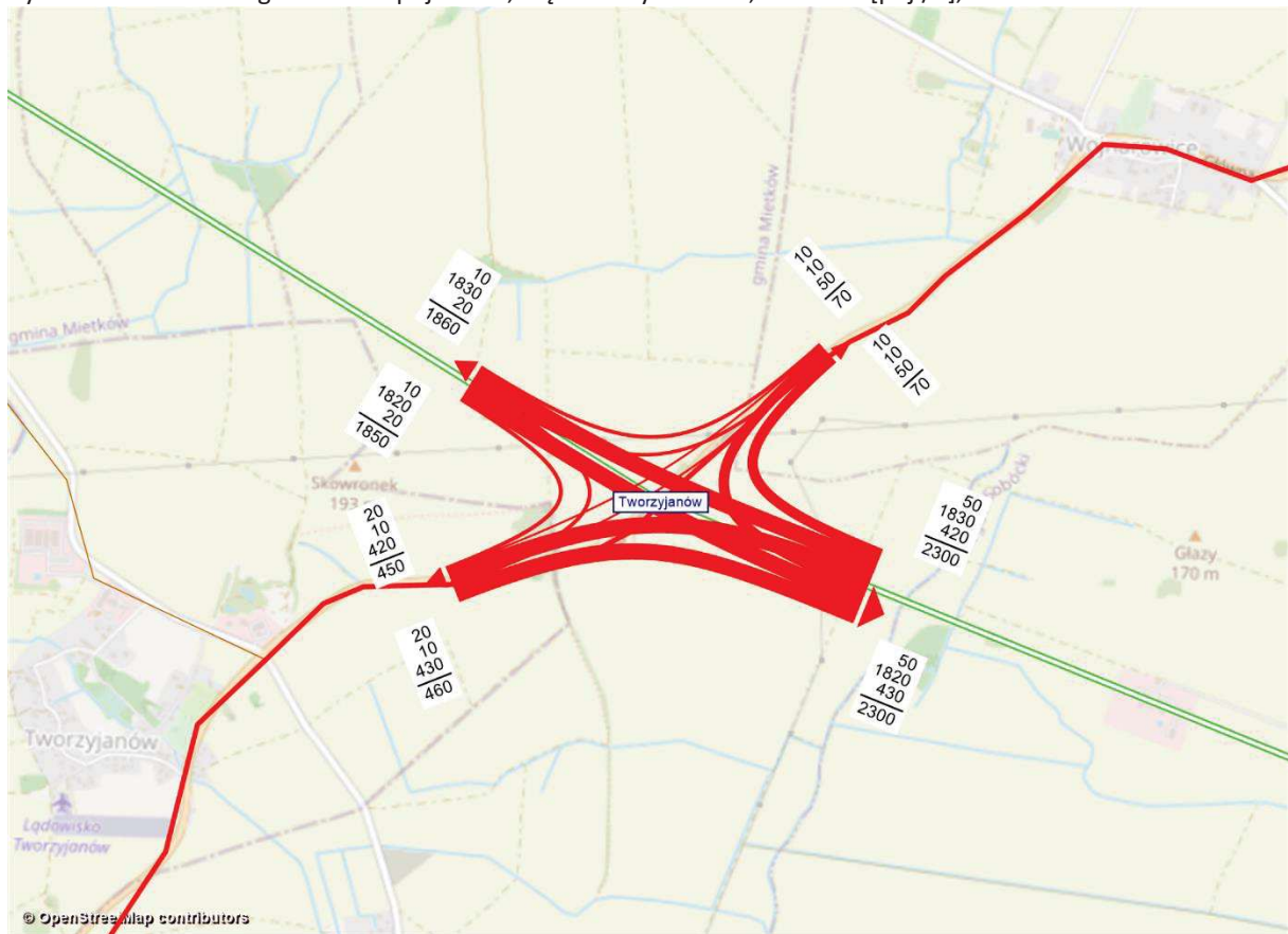
Rysunek 11.193 Kartogram ruchu pojazdów, węzeł Tworzyjanów, rok 2030 [poj./h], wariant W2WII
