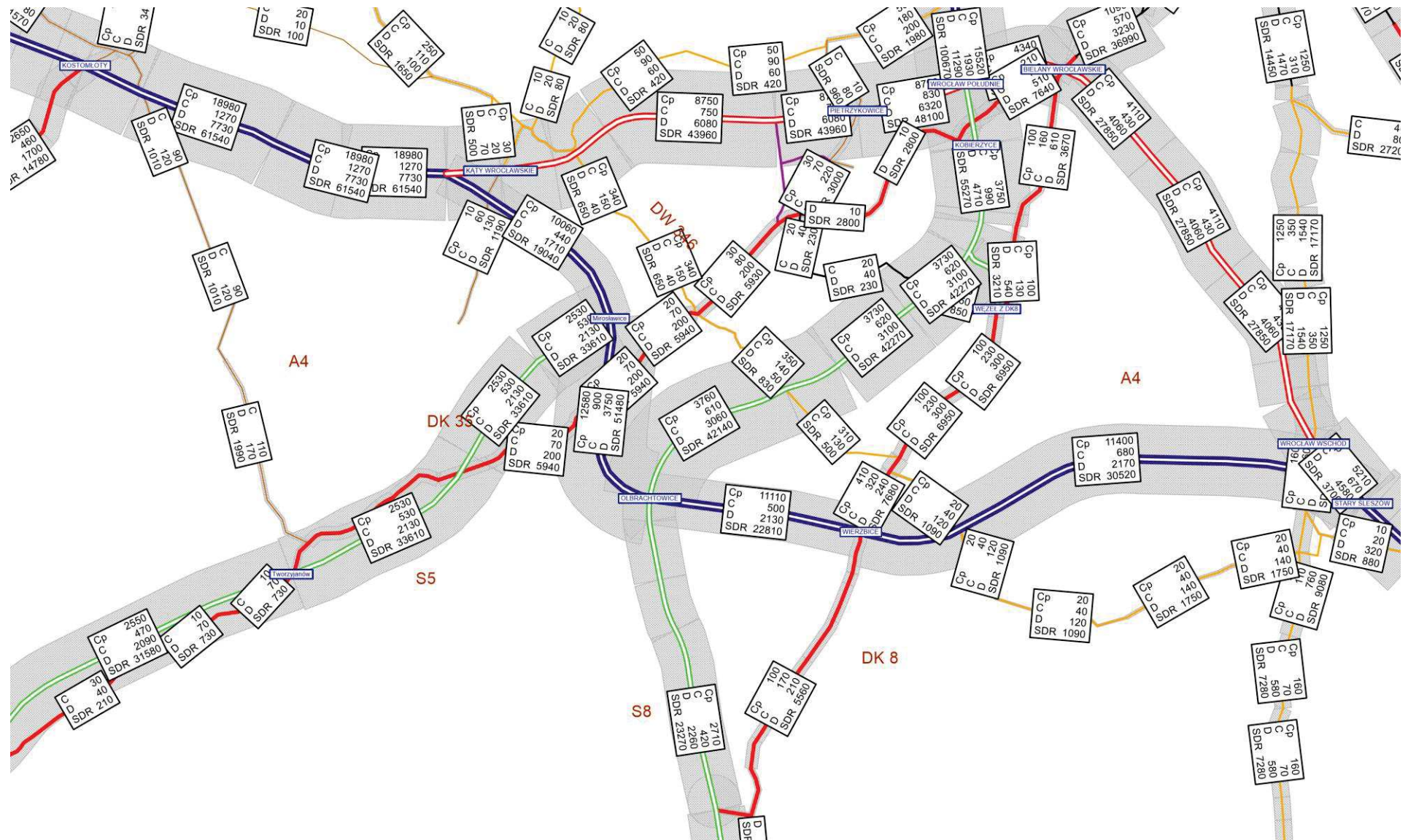
Rysunek 11.92 Natężenie pojazdów SDRR [poj./dobę], rok 2030 – W2.1WI , rys 2
