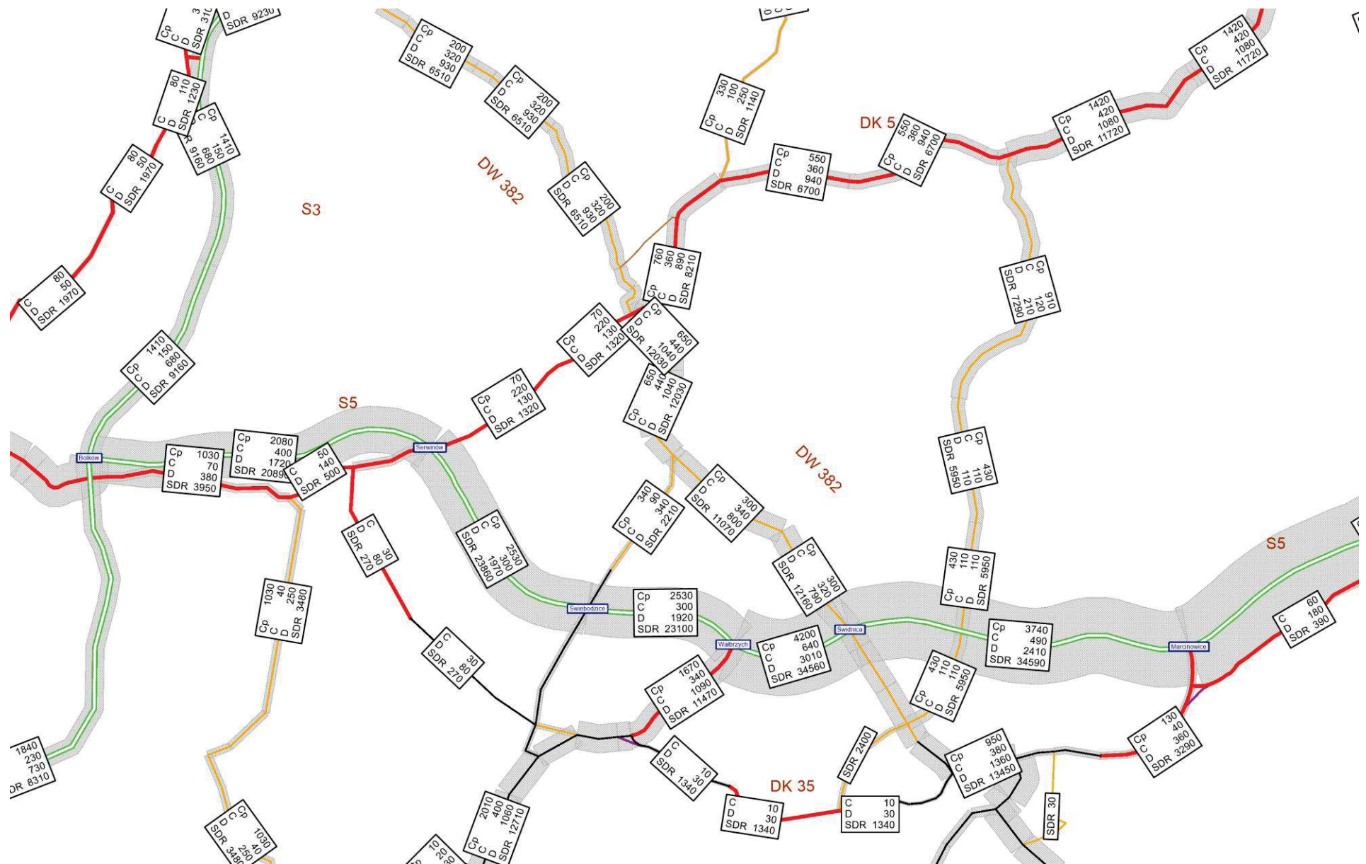
Rysunek 11.108 Natężenie pojazdów SDRR [poj./dobę], rok 2030 – W2.1WII, rys 3
