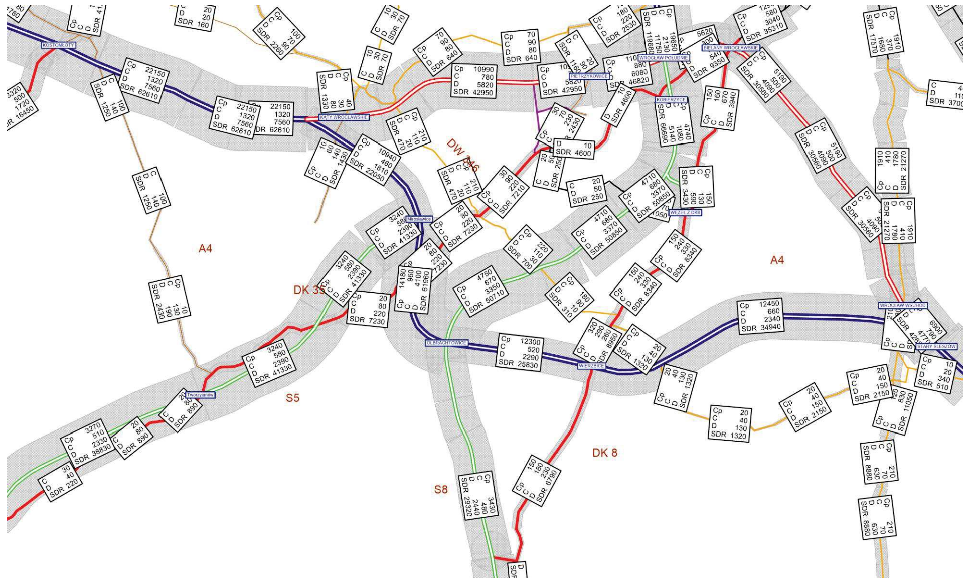
Rysunek 11.98 Natężenie pojazdów SDRR [poj./dobę], rok 2040 – W2.1WI, rys 2
