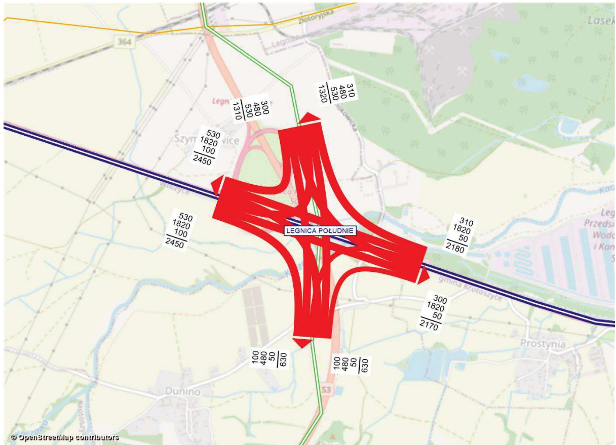
Rysunek 11.136 Kartogram ruchu pojazdów, węzeł Legnica Południe, rok 2030 [poj./h], wariant W1WII
