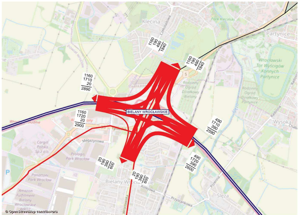
Rysunek 11.143 Kartogram ruchu pojazdów, węzeł Bielany Wrocławskie, rok 2030 [poj./h], wariant W1WII
