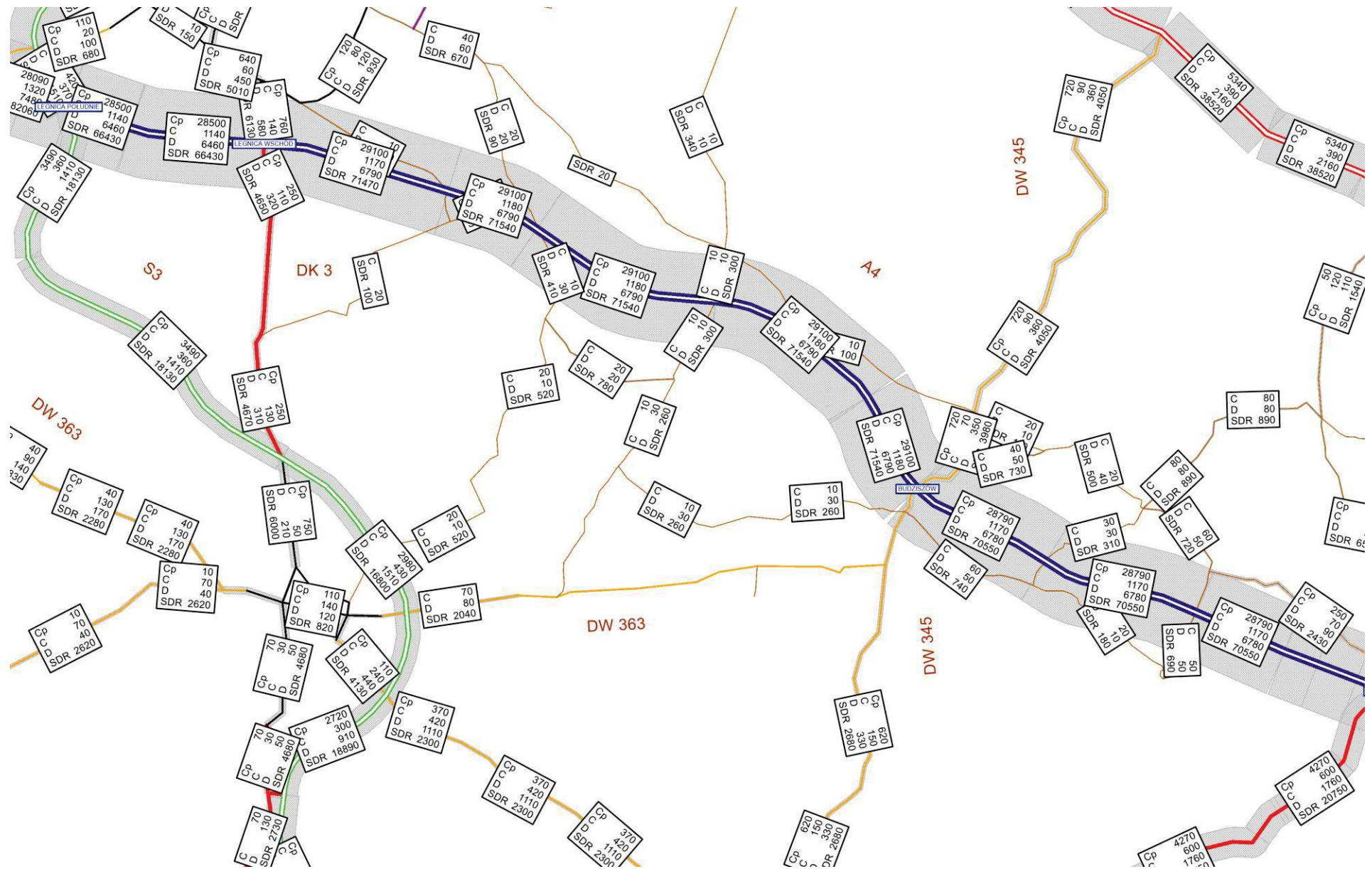
Rysunek 11.133 Natężenie pojazdów SDRR [poj./dobę], rok 2060 – W2.1WIII, rys 1
