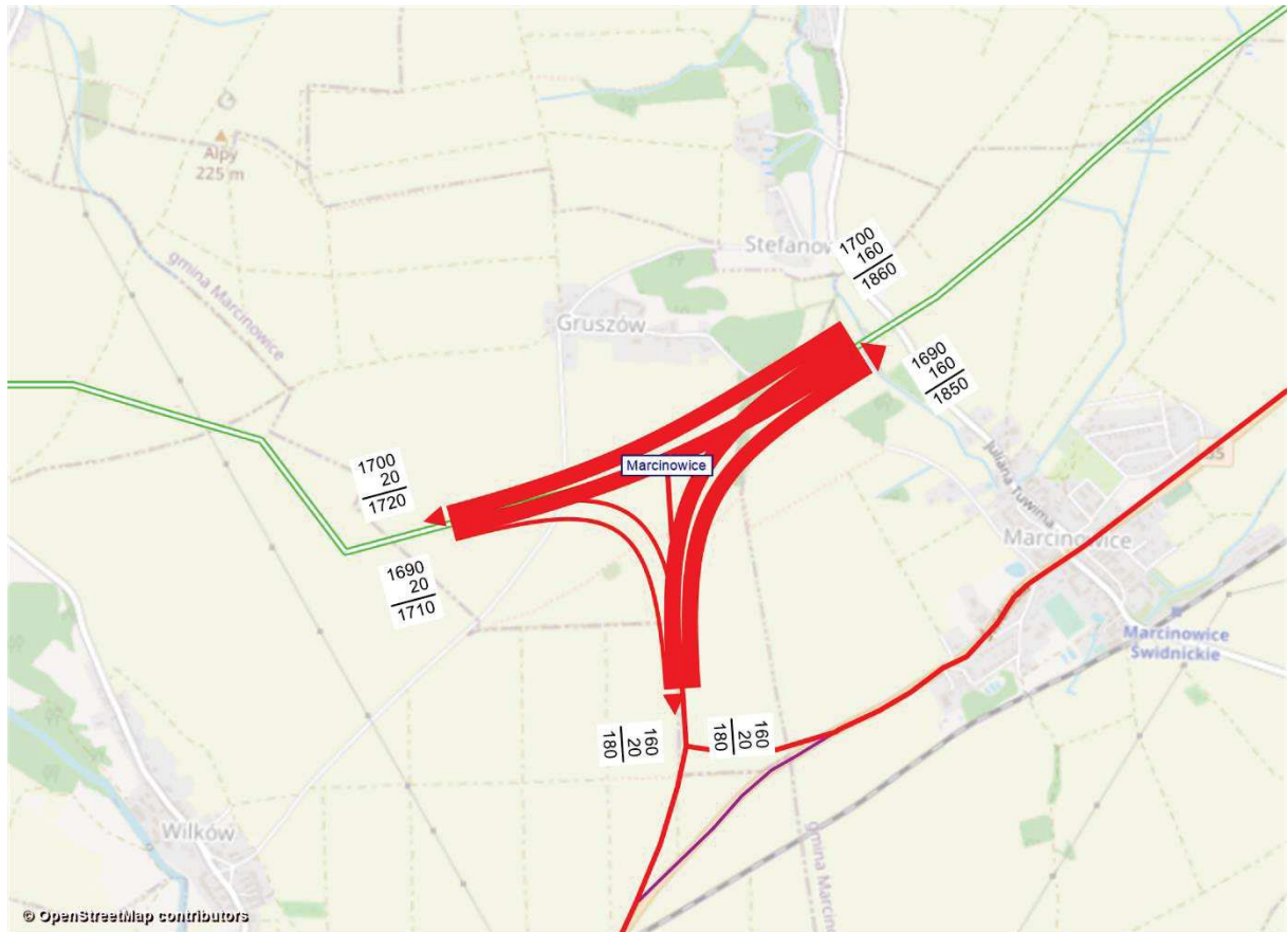
Rysunek 11.194 Kartogram ruchu pojazdów, węzeł Marcinowice, rok 2030 [poj./h], wariant W2WII
