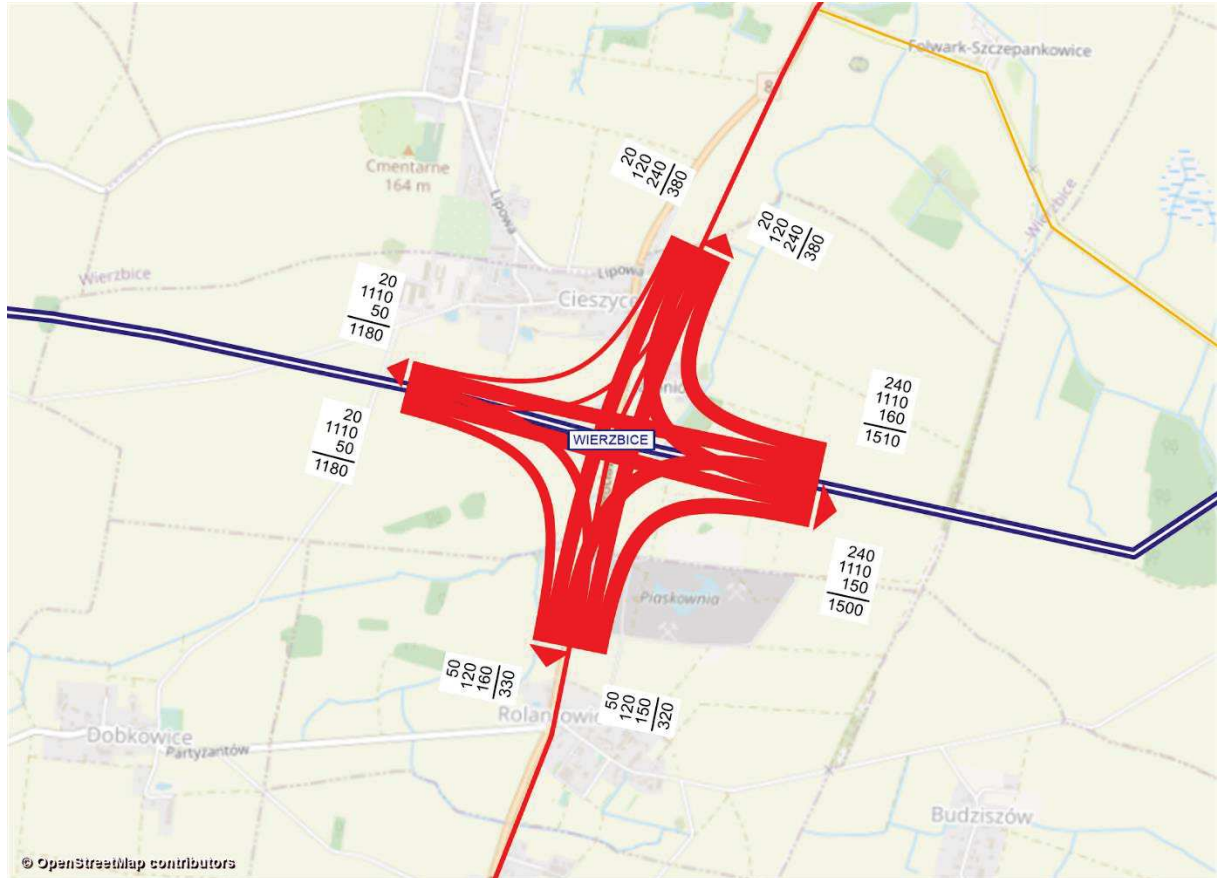
Rysunek 11.176 Kartogram ruchu pojazdów, węzeł Wierzbice, rok 2030 [poj./h], wariant W2WI
