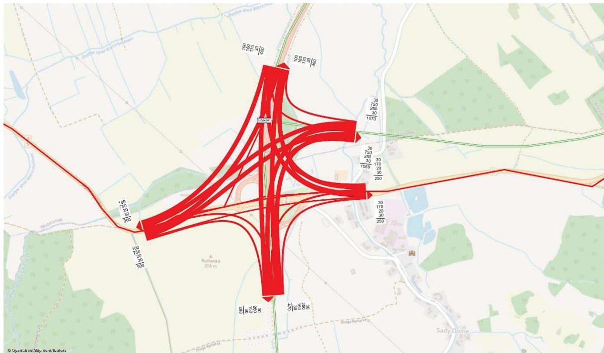
Rysunek 11.199 Kartogram ruchu pojazdów, węzeł Bolków, rok 2030 [poj./h], wariant W2WII
