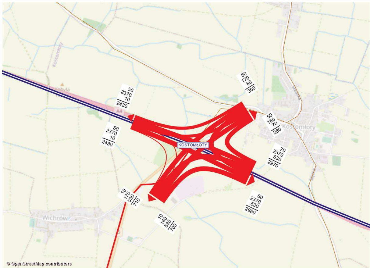
Rysunek 11.139 Kartogram ruchu pojazdów, węzeł Kostomłoty, rok 2030 [poj./h], wariant W1WII
