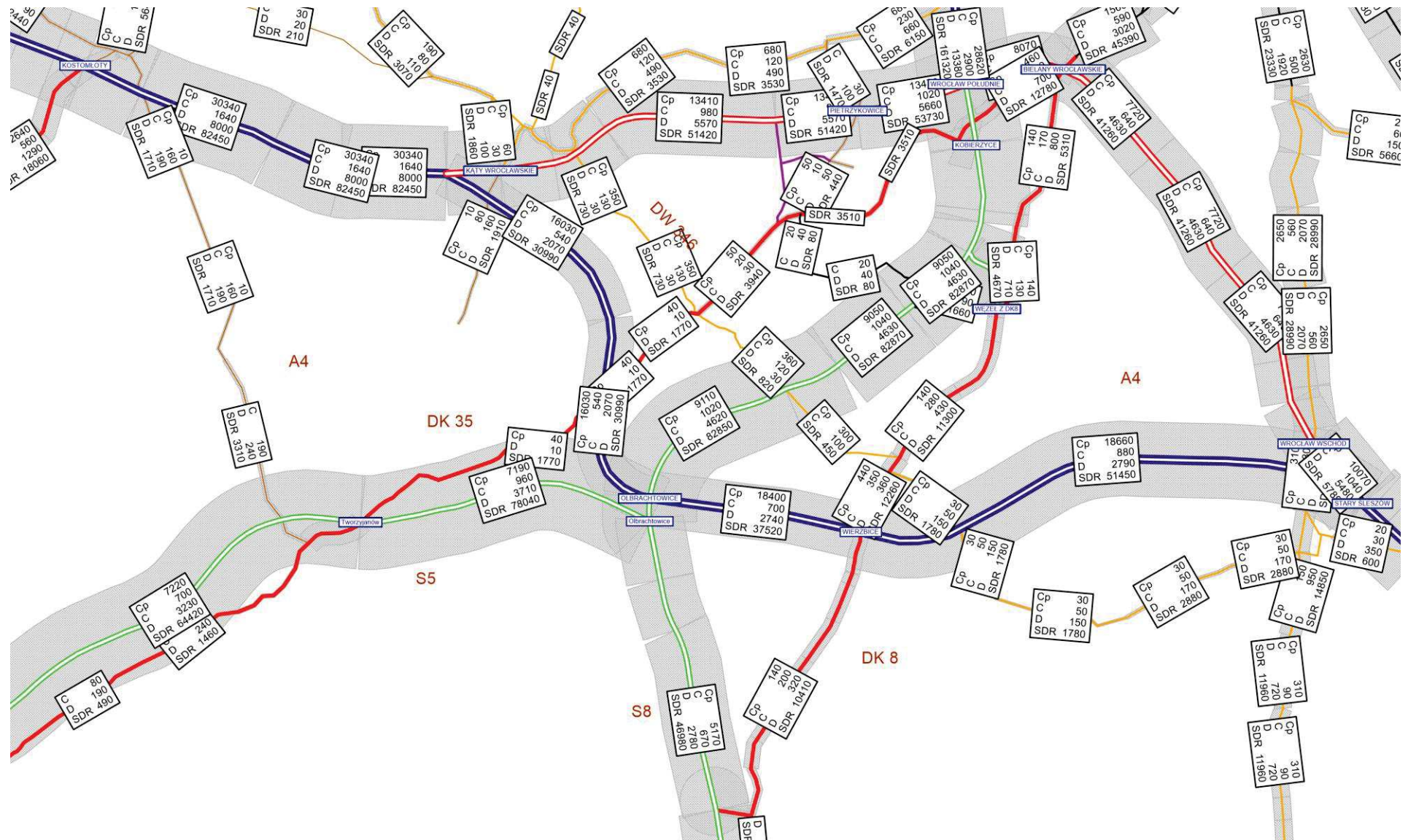
Rysunek 11.119 Natężenie pojazdów SDRR [poj./dobę], rok 2060 – W2.1WII, rys 2
