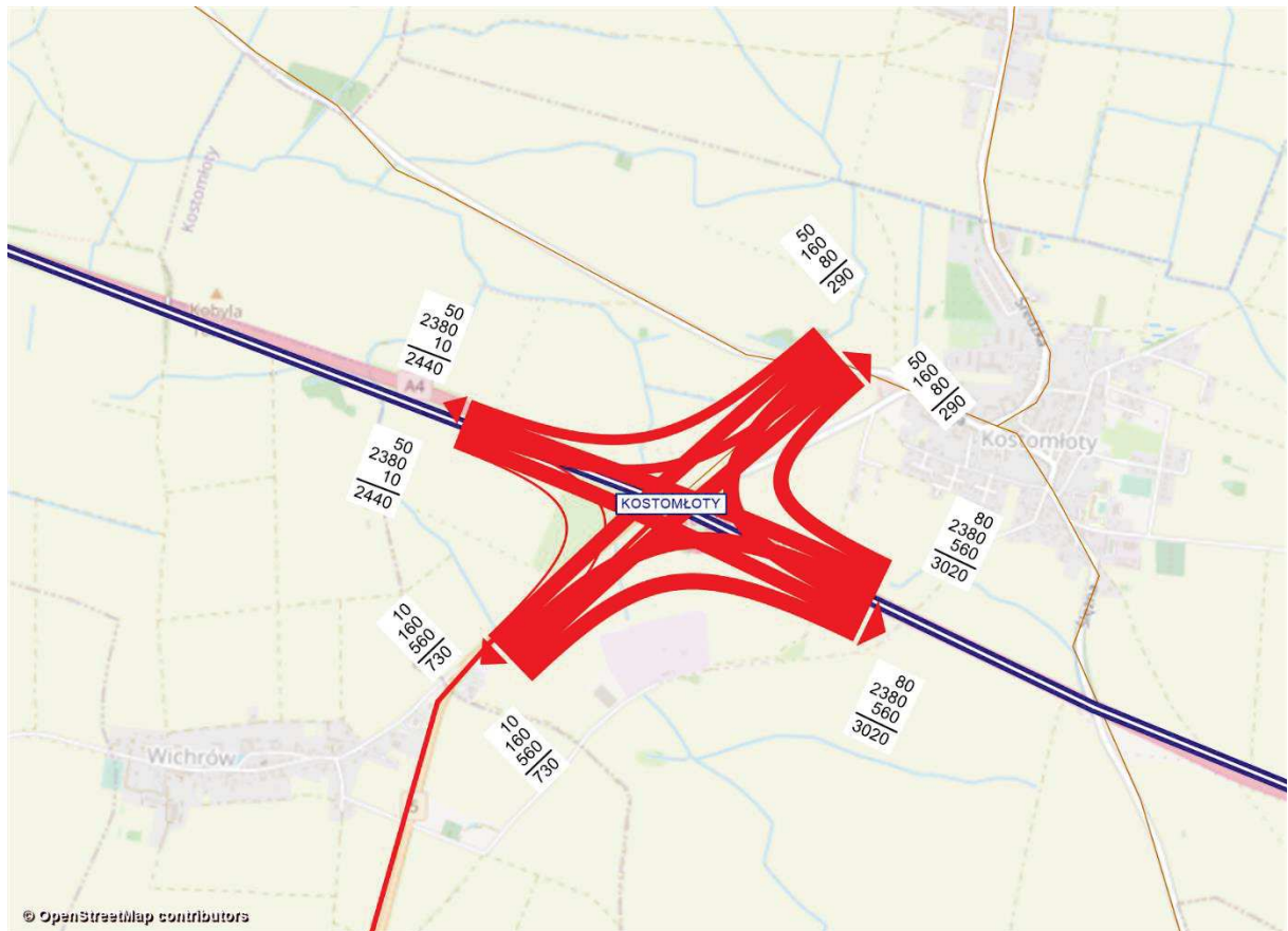
Rysunek 11.218 Kartogram ruchu pojazdów, węzeł Kostomłoty, rok 2030 [poj./h], wariant W2.1WI
