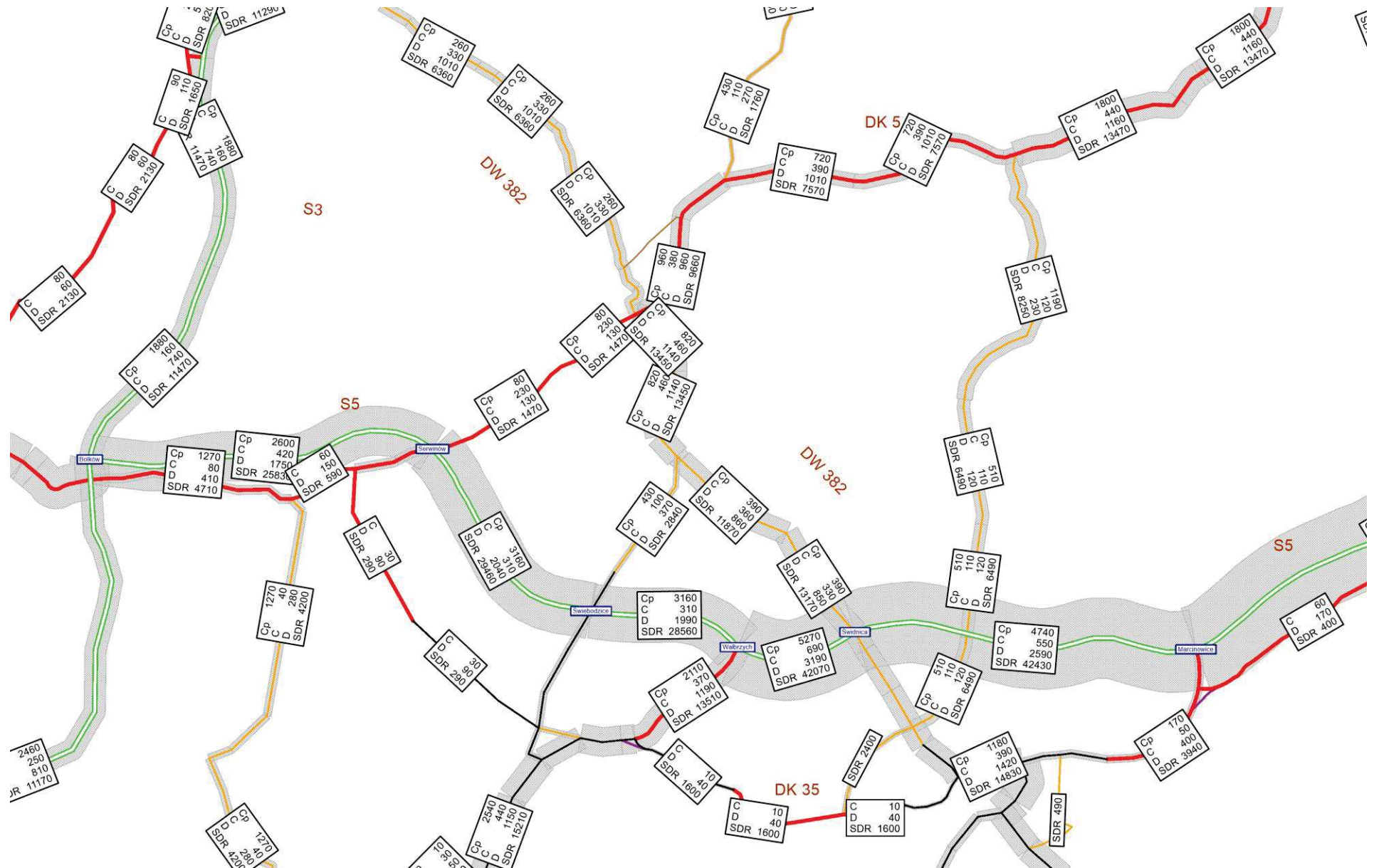
Rysunek 11.114 Natężenie pojazdów SDRR [poj./dobę], rok 2040 – W2.1WII, rys 3
