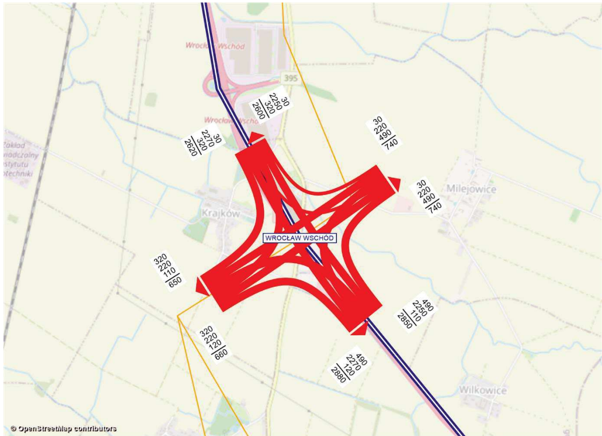
Rysunek 11.161 Kartogram ruchu pojazdów, węzeł Wrocław Wschód, rok 2030 [poj./h], wariant W1WIII
