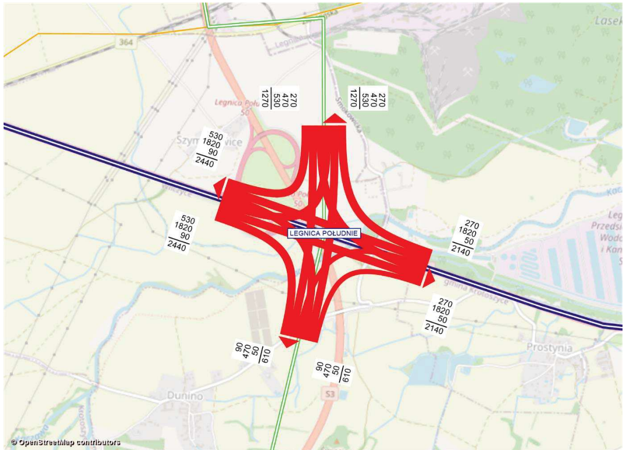
Rysunek 11.186 Kartogram ruchu pojazdów, węzeł Legnica Południe, rok 2030 [poj./h], wariant W2WII
