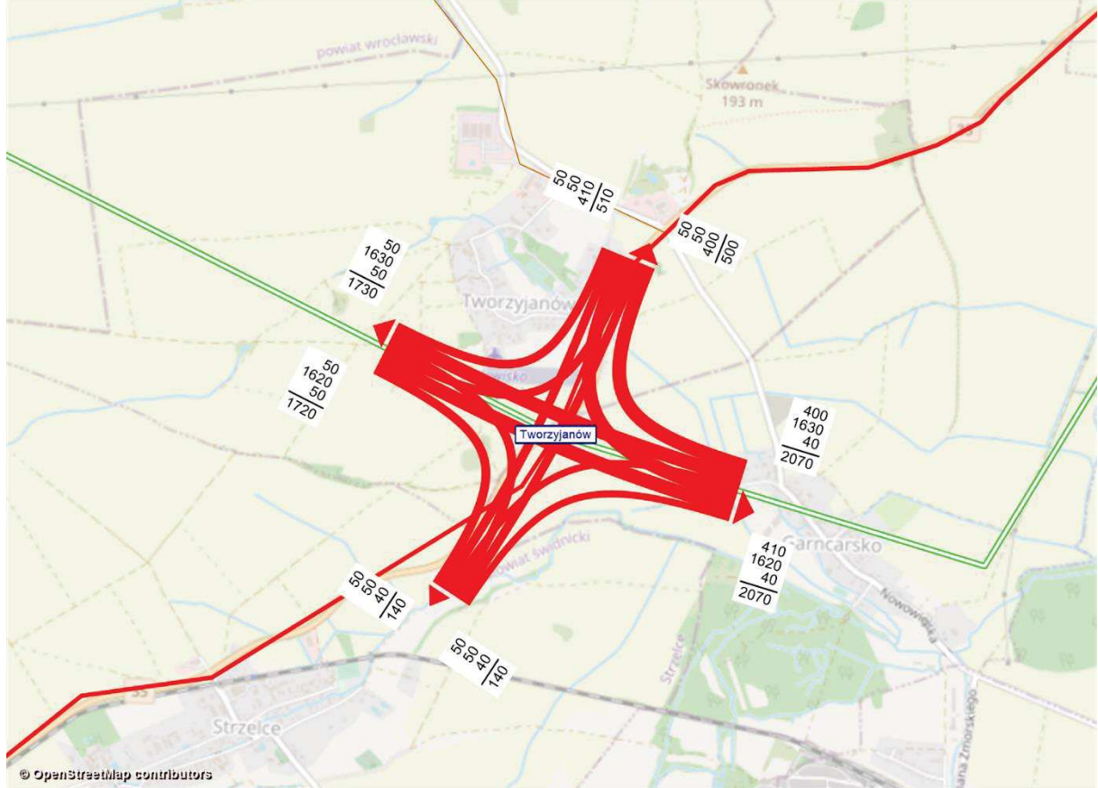
Rysunek 11.179 Kartogram ruchu pojazdów, węzeł Tworzyjanów, rok 2030 [poj./h], wariant W2W1
