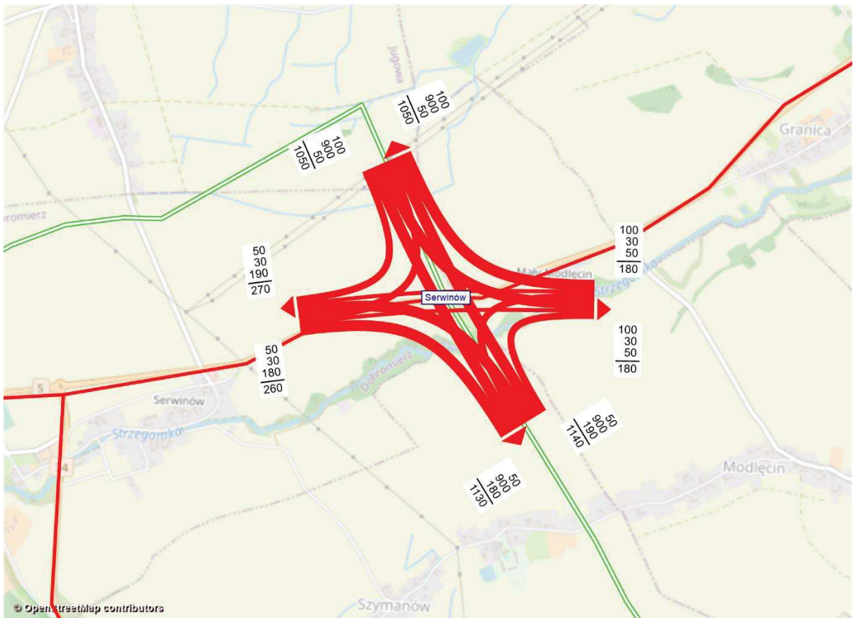
Rysunek 11.230 Kartogram ruchu pojazdów, węzeł Serwinów, rok 2030 [poj./h], wariant W2.1WI
