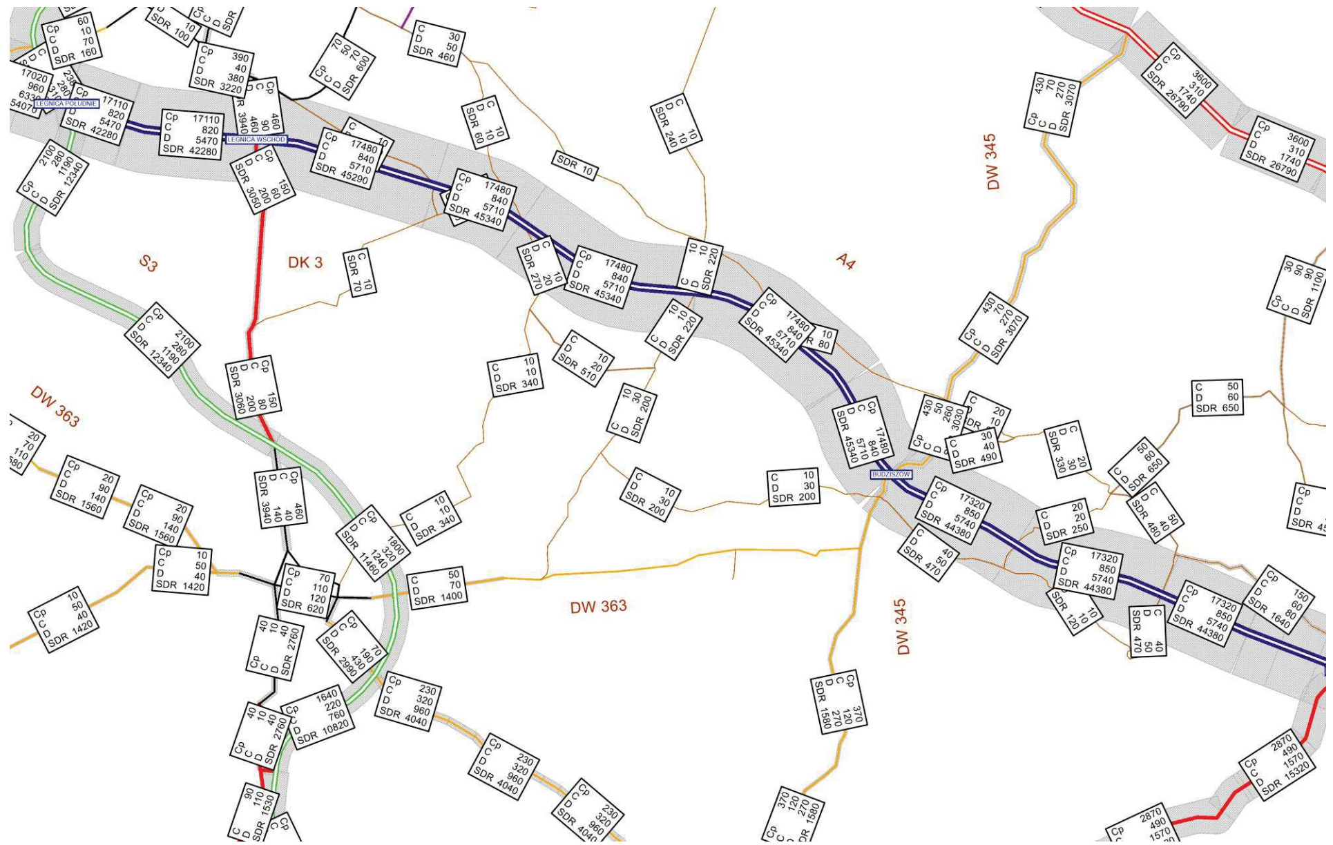
Rysunek 11.124 Natężenie pojazdów SDRR [poj./dobę], rok 2035 – W2.1WIII, rys 1
