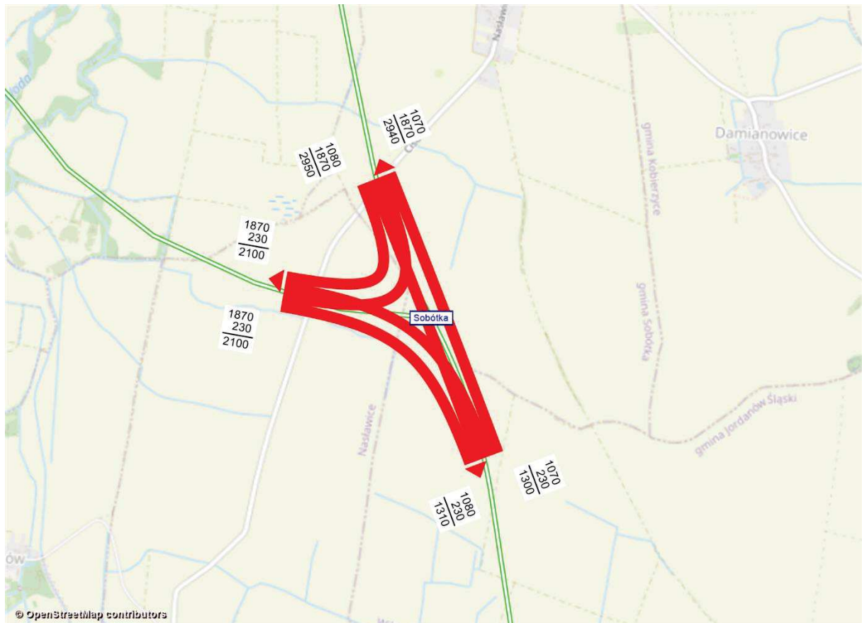
Rysunek 11.207 Kartogram ruchu pojazdów, węzeł Sobótka, rok 2030 [poj./h], wariant W2WIII
