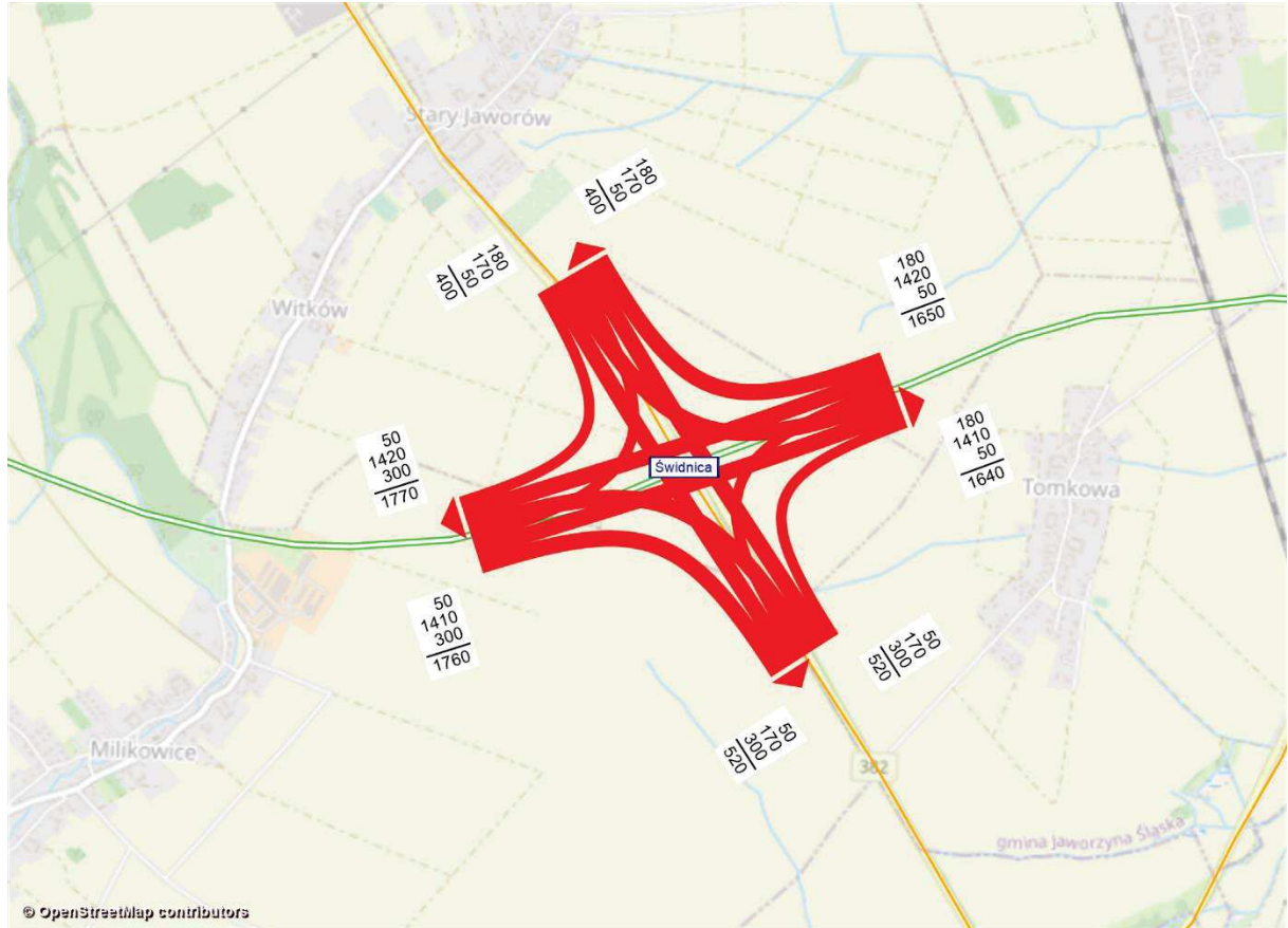
Rysunek 11.210 Kartogram ruchu pojazdów, węzeł Świdnica, rok 2030 [poj./h], wariant W2WIII
