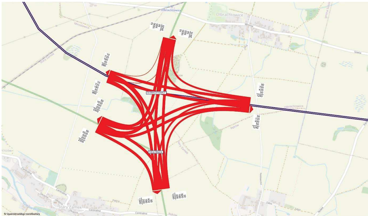
Rysunek 11.190 Kartogram ruchu pojazdów, węzeł Olbrachtowice, rok 2030 [poj./h], wariant W2WII
