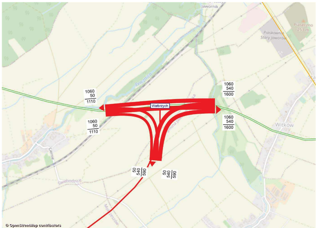
Rysunek 11.228 Kartogram ruchu pojazdów, węzeł Wałbrzych, rok 2030 [poj./h], wariant W2.1W1
