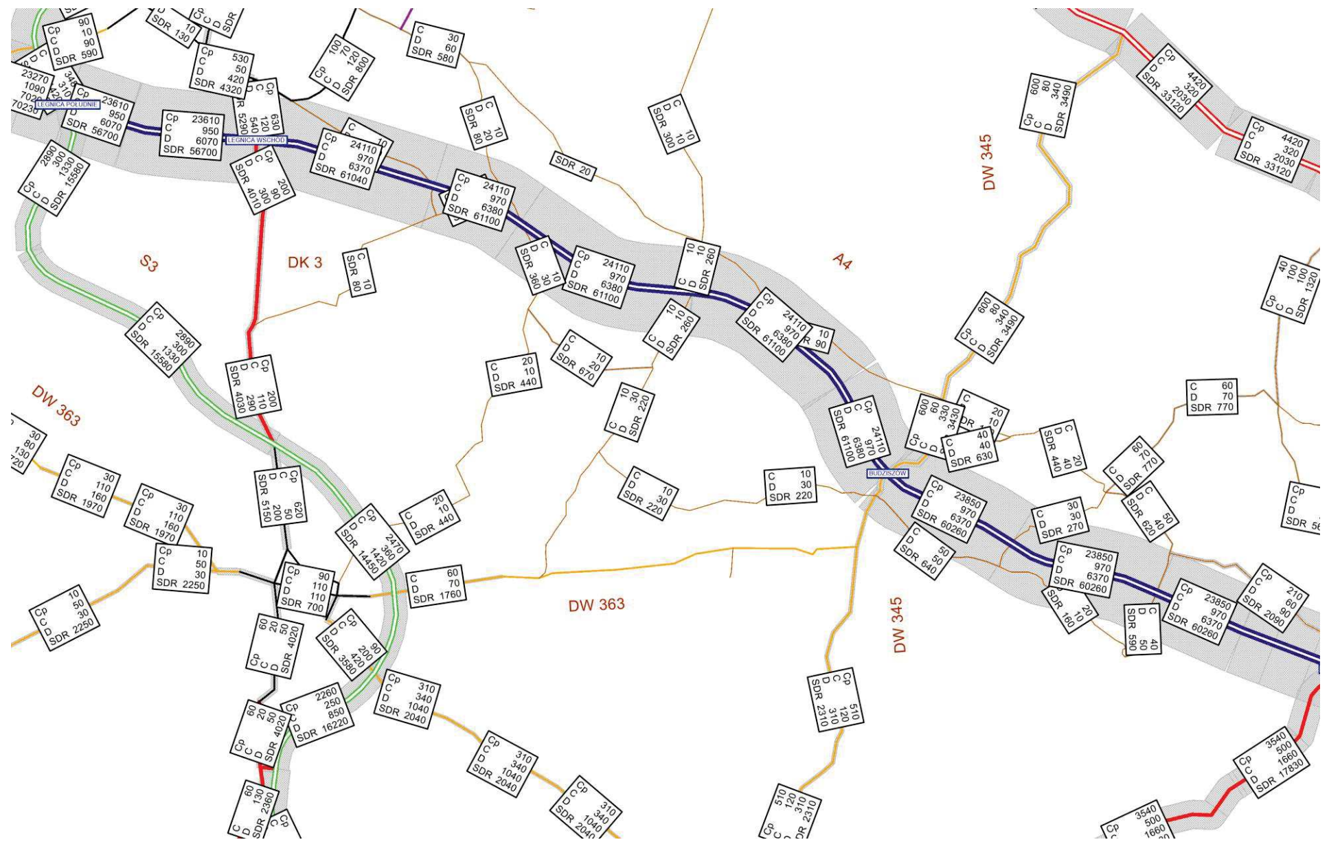
Rysunek 11.130 Natężenie pojazdów SDRR [poj./dobę], rok 2050 – W2.1WIII, rys 1
