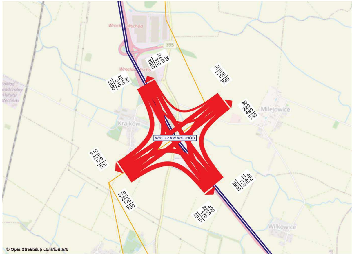
Rysunek 11.144 Kartogram ruchu pojazdów, węzeł Wrocław Wschód, rok 2030 [poj./h], wariant W1WII
