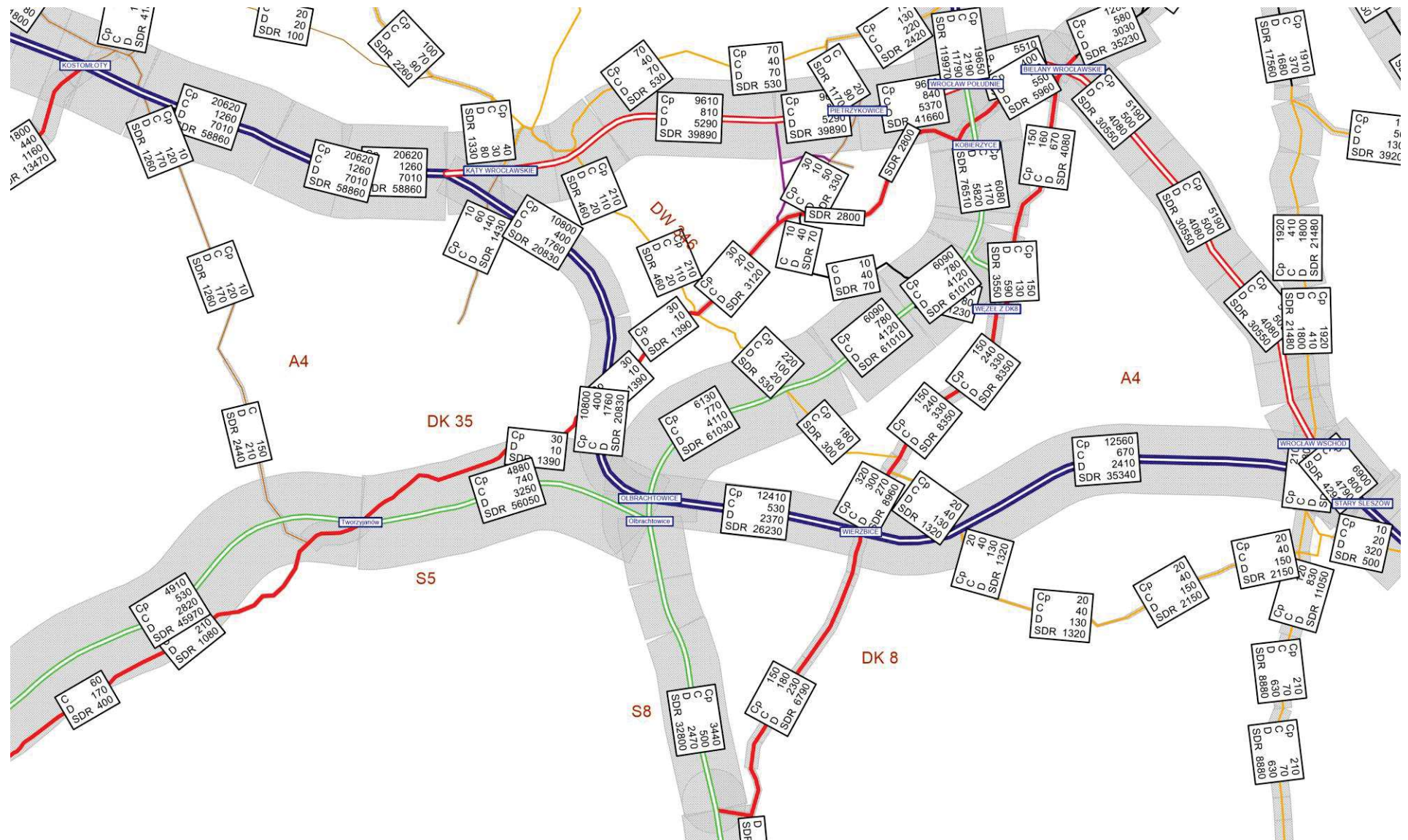
Rysunek 11.113 Natężenie pojazdów SDRR [poj./dobę], rok 2040 – W2.1WII, rys 2
