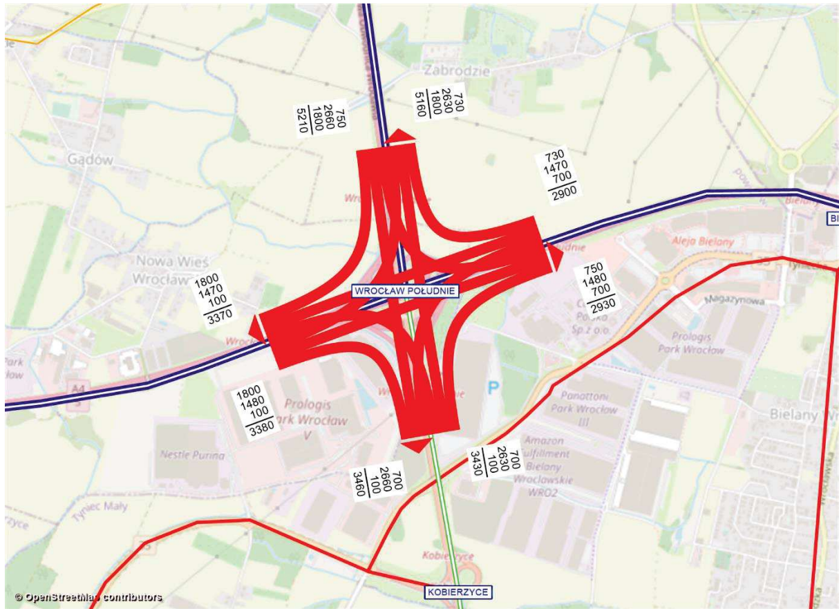
Rysunek 11.159 Kartogram ruchu pojazdów, węzeł Wrocław Południe, rok 2030 [poj./h], wariant W1WIII
