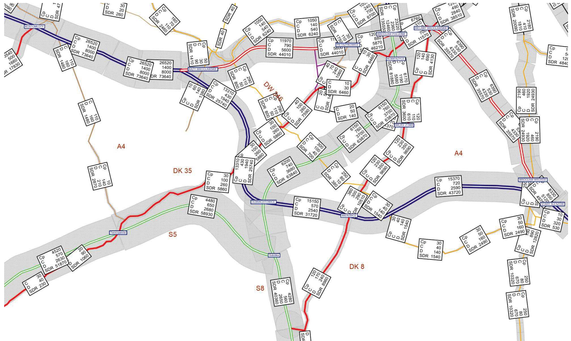
Rysunek 11.131 Natężenie pojazdów SDRR [poj./dobę], rok 2050 – W2.1WIII, rys 2
