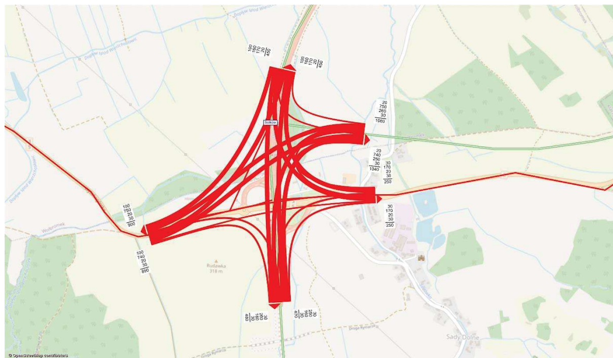
Rysunek 11.152 Kartogram ruchu pojazdów, węzeł Bolków, rok 2030 [poj./h], wariant W1WII
