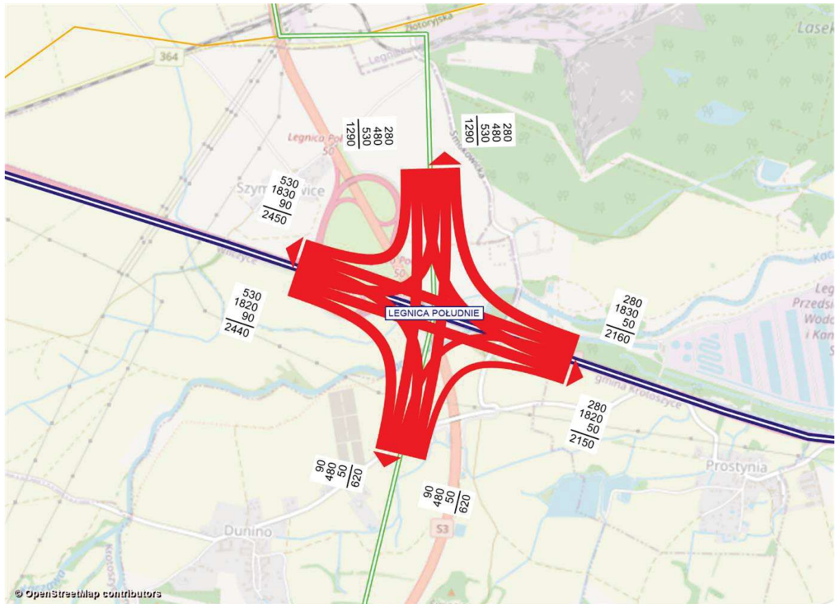
Rysunek 11.232 Kartogram ruchu pojazdów, węzeł Legnica Południe, rok 2030 [poj./h], wariant W2.1WII
