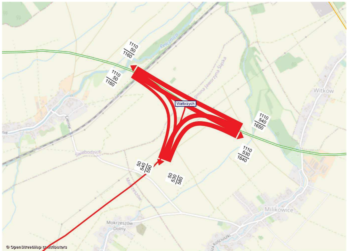
Rysunek 11.166 Kartogram ruchu pojazdów, węzeł Wałbrzych, rok 2030 [poj./h], wariant W1WIII
