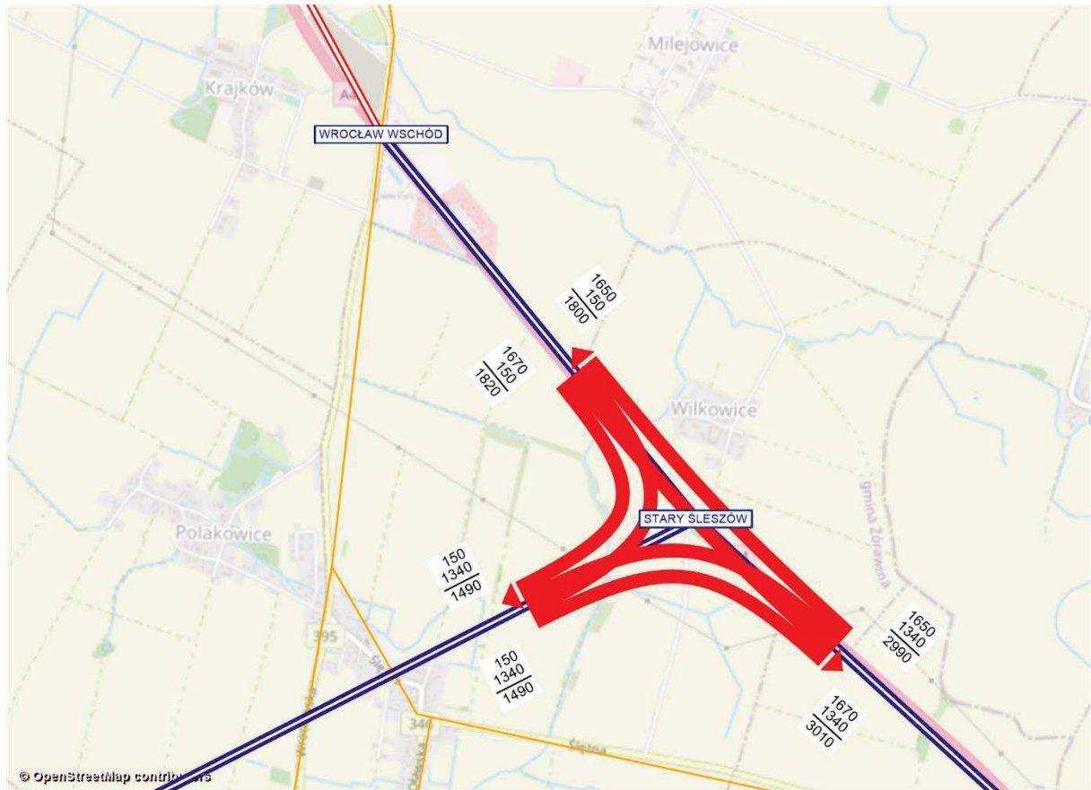
Rysunek 11.223 Kartogram ruchu pojazdów, węzeł Stary Sleszów, rok 2030 [poj./h], wariant W2.1WI
