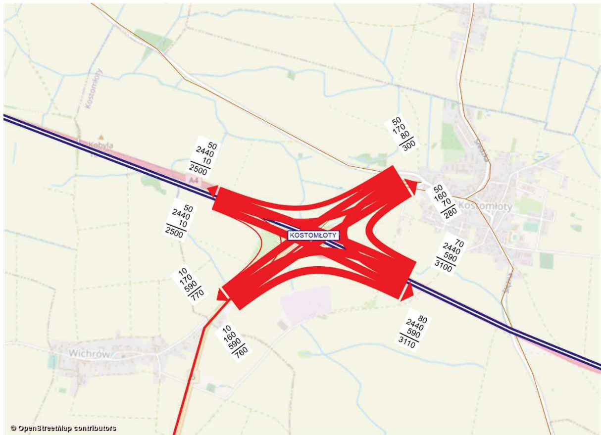
Rysunek 11.156 Kartogram ruchu pojazdów, węzeł Kostomłoty, rok 2030 [poj./h], wariant W1WIII
