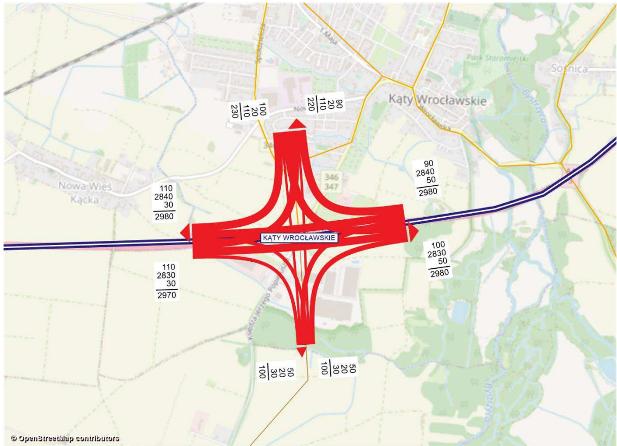
Rysunek 11.140 Kartogram ruchu pojazdów, węzeł Kąty Wrocławskie, rok 2030 [poj./h], wariant W1WII
