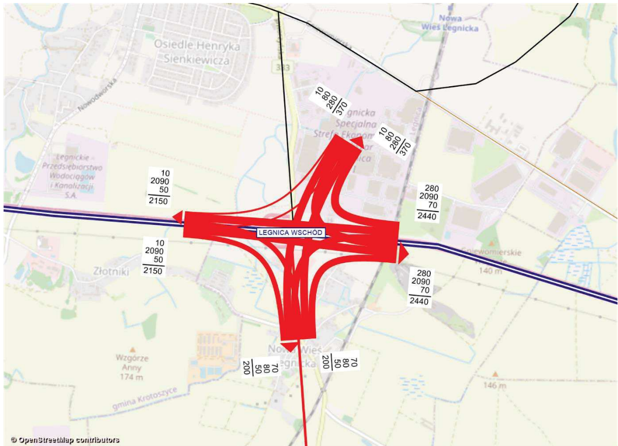
Rysunek 11.216 Kartogram ruchu pojazdów, węzeł Legnica Wschód, rok 2030 [poj./h], wariant W2.1W1
