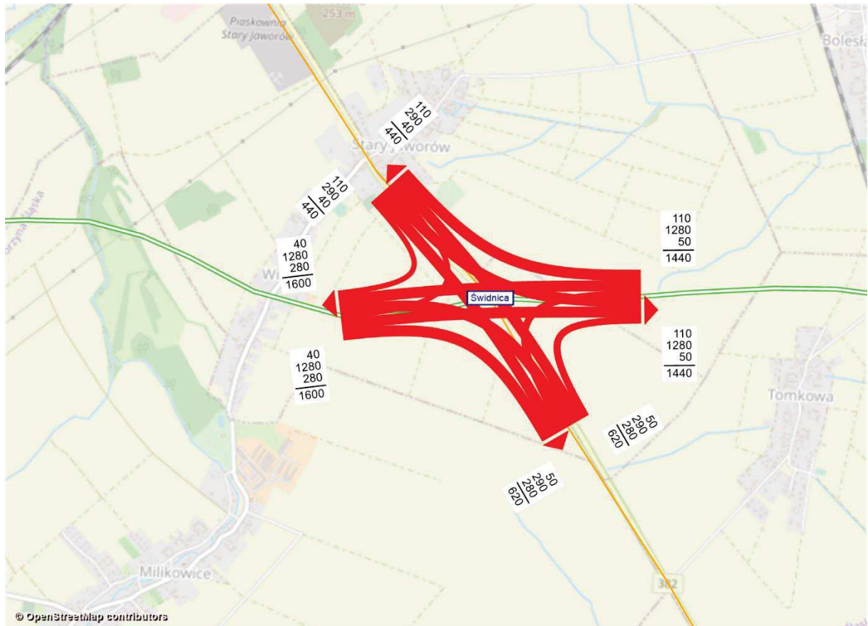
Rysunek 11.227 Kartogram ruchu pojazdów, węzeł Świdnica, rok 2030 [poj./h], wariant W2.1W1
