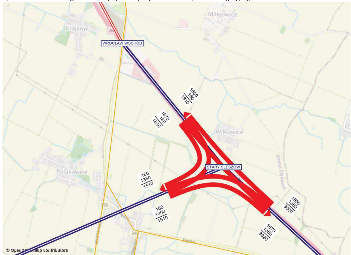
Rysunek 11.177 Kartogram ruchu pojazdów, węzeł Stary Sleszów, rok 2030 [poj./h], wariant W2WI
