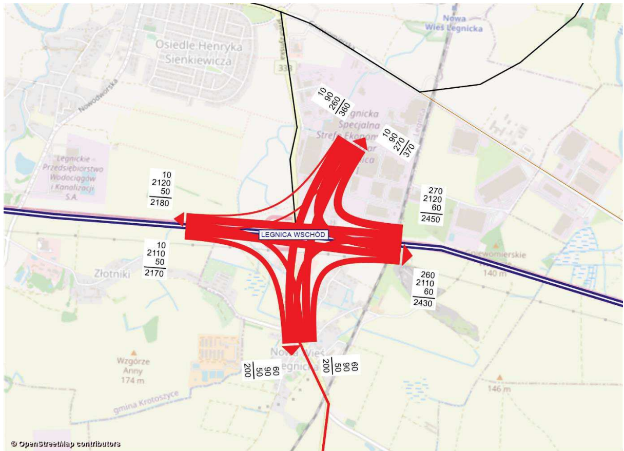
Rysunek 11.137 Kartogram ruchu pojazdów, węzeł Legnica Wschód, rok 2030 [poj./h], wariant W1WII
