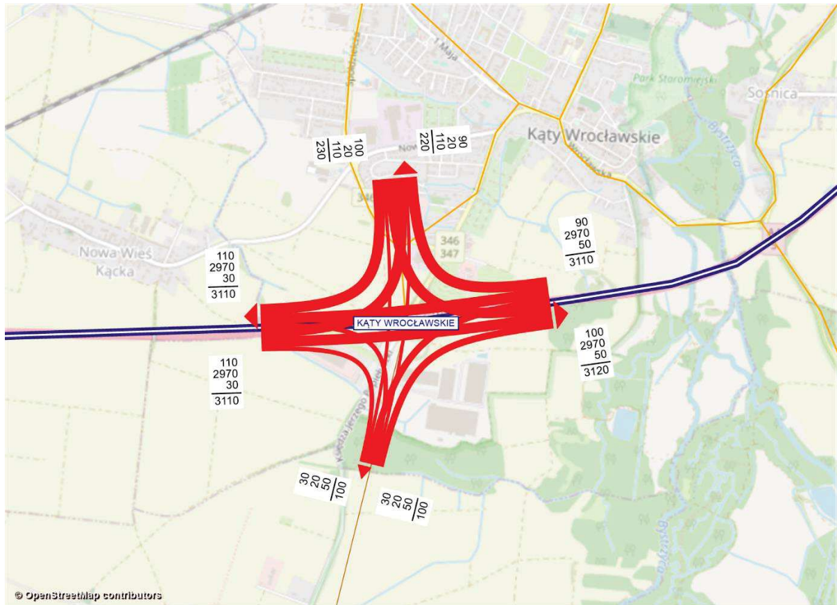
Rysunek 11.157 Kartogram ruchu pojazdów, węzeł Kąty Wrocławskie, rok 2030 [poj./h], wariant W1WIII
