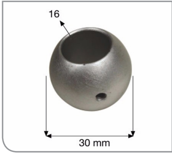
Ürün Kodu: 3045-b 16'lik Boru Süsü (Çap 30)
