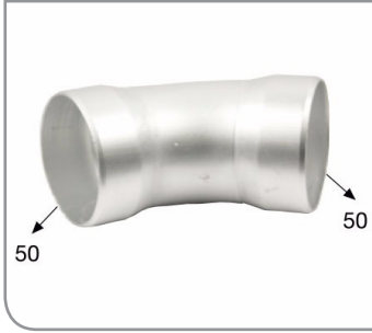
Ürün Kodu: 2684-a / b / c / d 50'lik - 40'lik - 35'lik - 30'lik Dirsek 135° 1/8 Bilezikli (İçi Boş)
