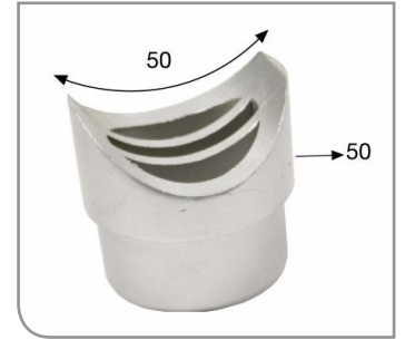
Ürün Kodu: 2719 50'lik Boru İçin 50'lik Kurtağız
