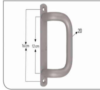
Ürün Kodu: 1611 Aynalı Kıvrık Çekme Kol
