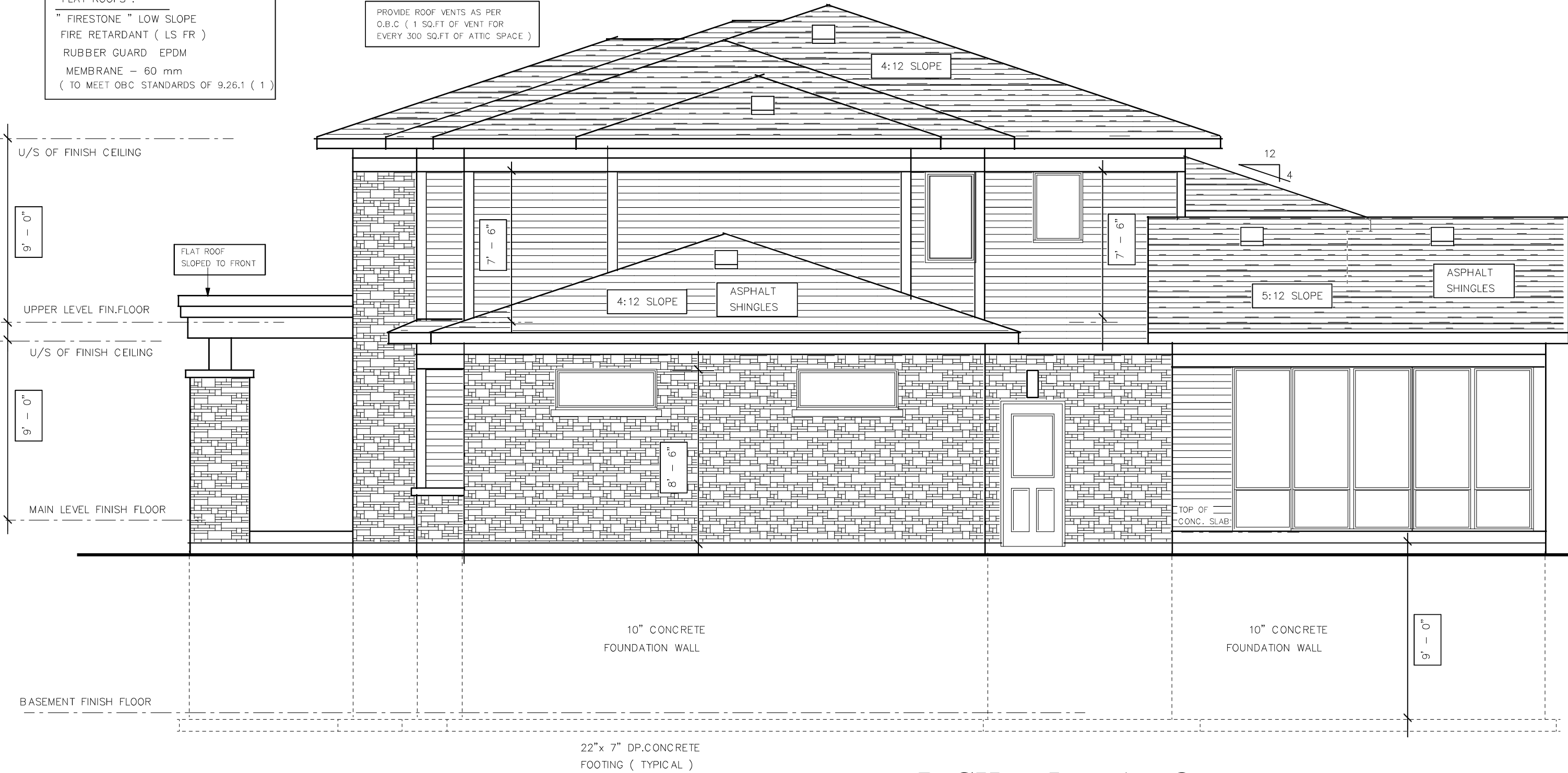
RIGHT ELEVATION
