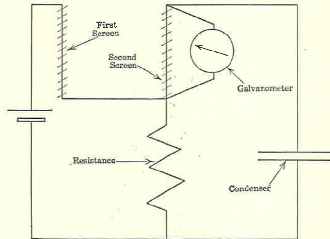
FIG. 48. Condenser Chronoscope.
