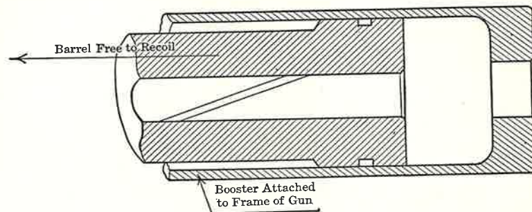
FIG. 22. Muzzle Booster.
