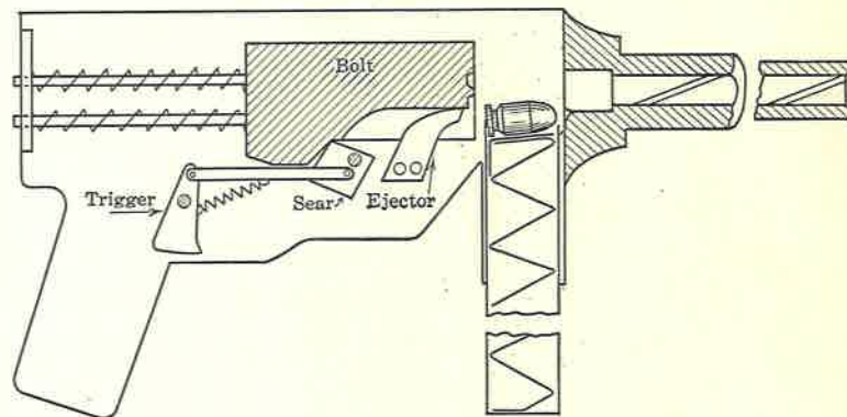
FIG. 24. U. S. Submachine Gun, Cal. .45, M3.
