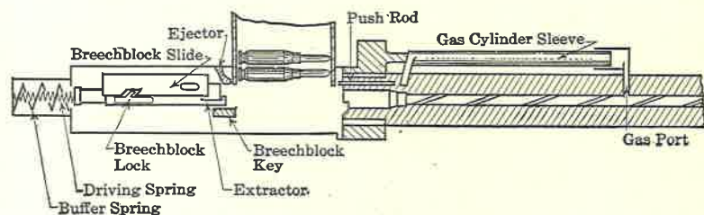
FIG. 31. Hispano-Suiza 20 mm Automatic Cannon.
