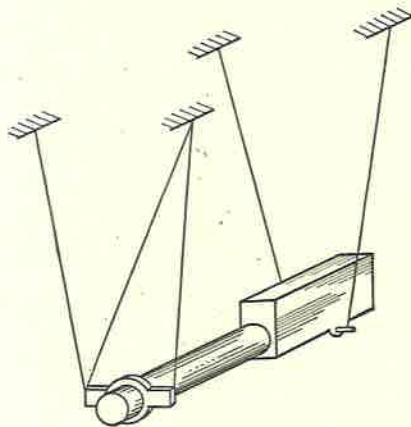
FIG. 51. Ballistic Pendulum.
