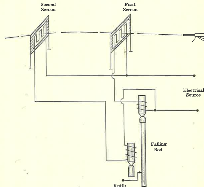
FIG. 47. Boulengé Chronograph.
