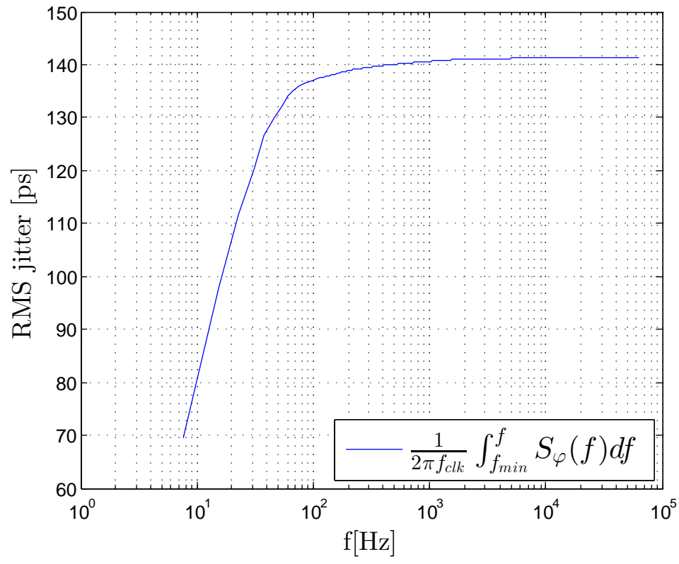
Jitter - warto skuteczna
